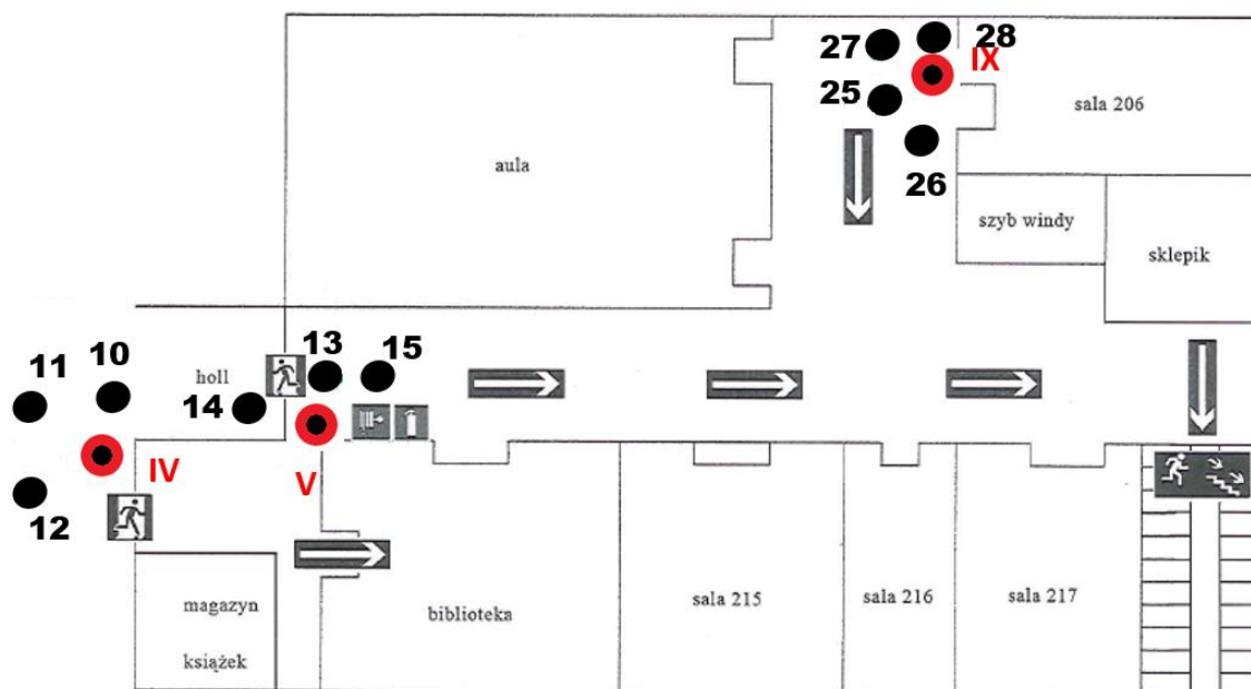
Rys. 1c: Plan rozmieszczenia punktów pomiarowych – I piętro część 1 kolorem czerwonym oznaczono lokalizację punktów dostępowych
