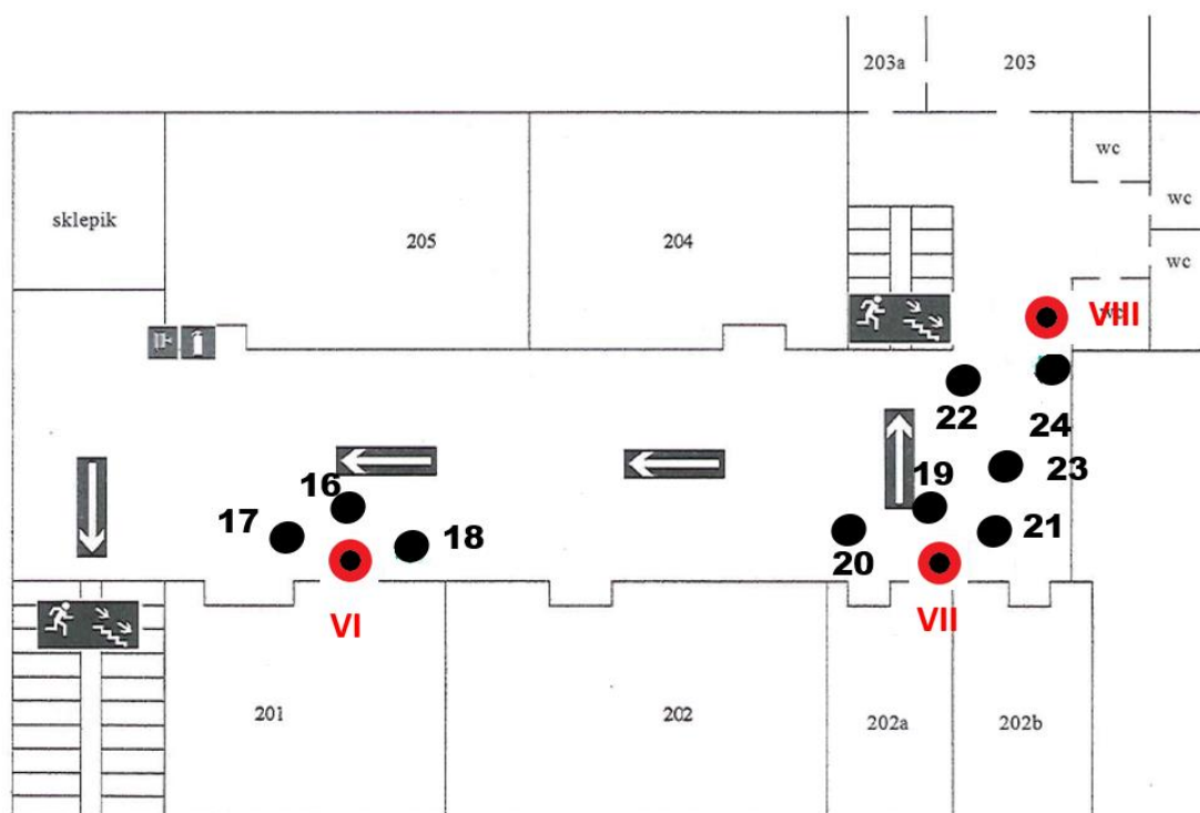
Rys. 1c: Plan rozmieszczenia punktów pomiarowych – I piętro część 1 kolorem czerwonym oznaczono lokalizację punktów dostępowych
