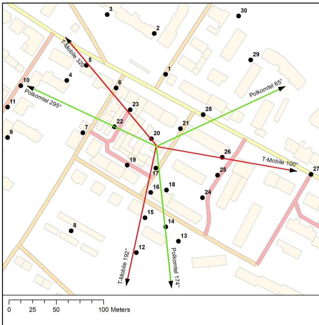
Rys. 1: Plan terenu, na którym znajdują się badane stacje bazowe
