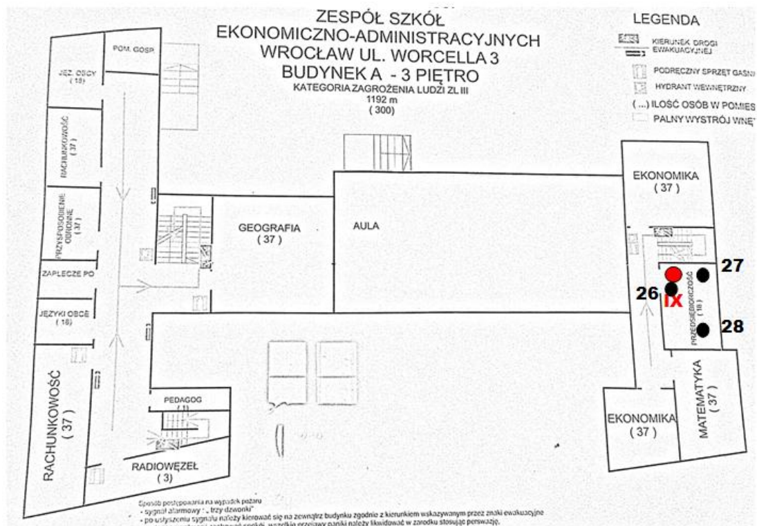
Rys. 1d: Plan rozmieszczenia punktów pomiarowych – III piętro, kolorem czerwonym oznaczono lokalizację punktów dostępowych
