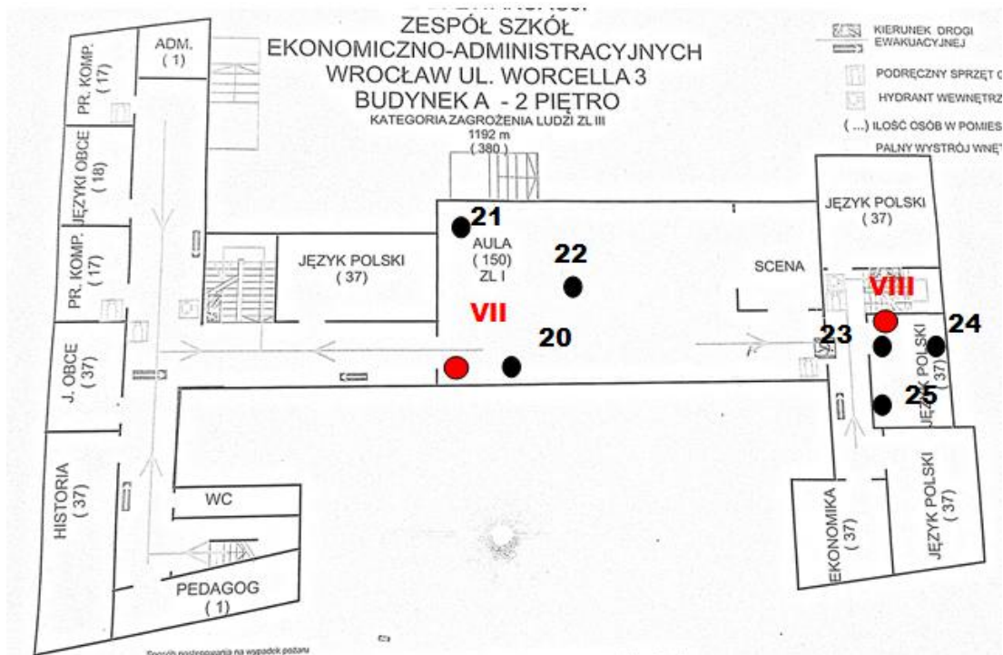
Rys. 1c: Plan rozmieszczenia punktów pomiarowych – II piętro, kolorem czerwonym oznaczono lokalizację punktów dostępowych
