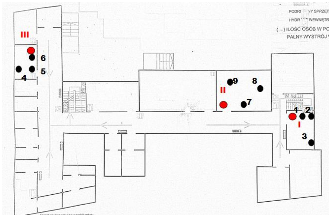
Rys. 1a: Plan rozmieszczenia punktów pomiarowych – parter, kolorem czerwonym oznaczono lokalizację punktów dostępnych
