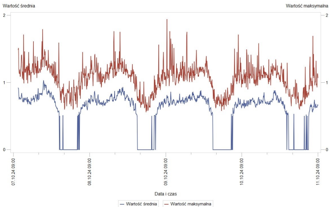
Rys. 6 Wyniki pomiarów – ZSO nr 1 w Mielcu w dniach 7.10.2024 r. – 11.10.2024 r. – wartość średnia i wartość maksymalna
