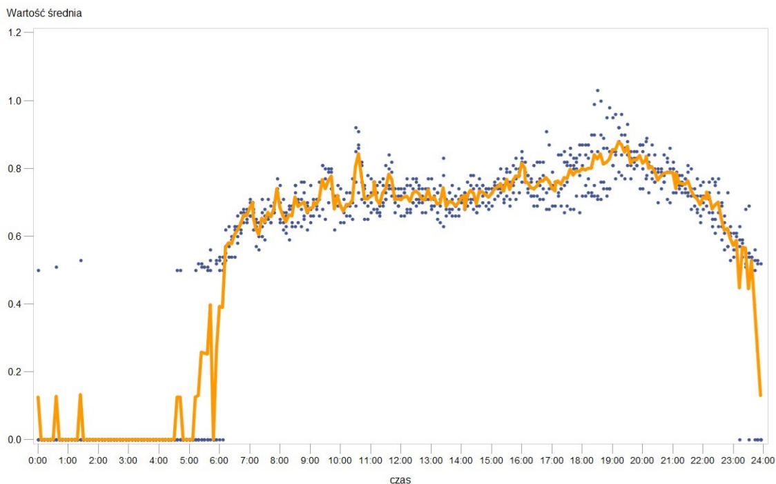
Rys. 7 Wyniki pomiarów – ZSO nr 1 w Mielcu – średnia za okres 24 godzin
