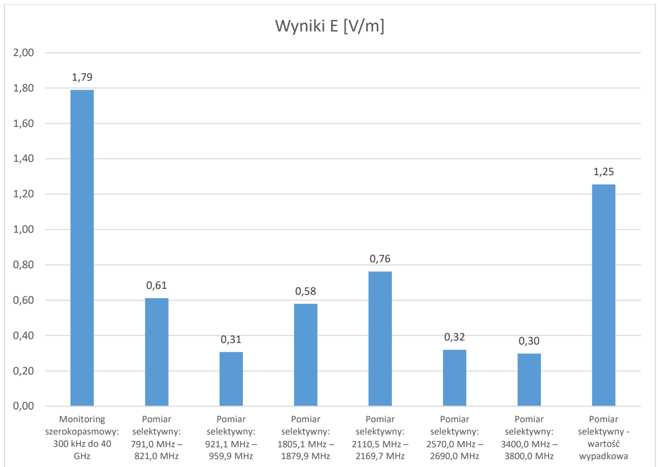
Rys. 15 Porównanie wyników monitoringu szerokopasmowego i pomiarów selektywnych
