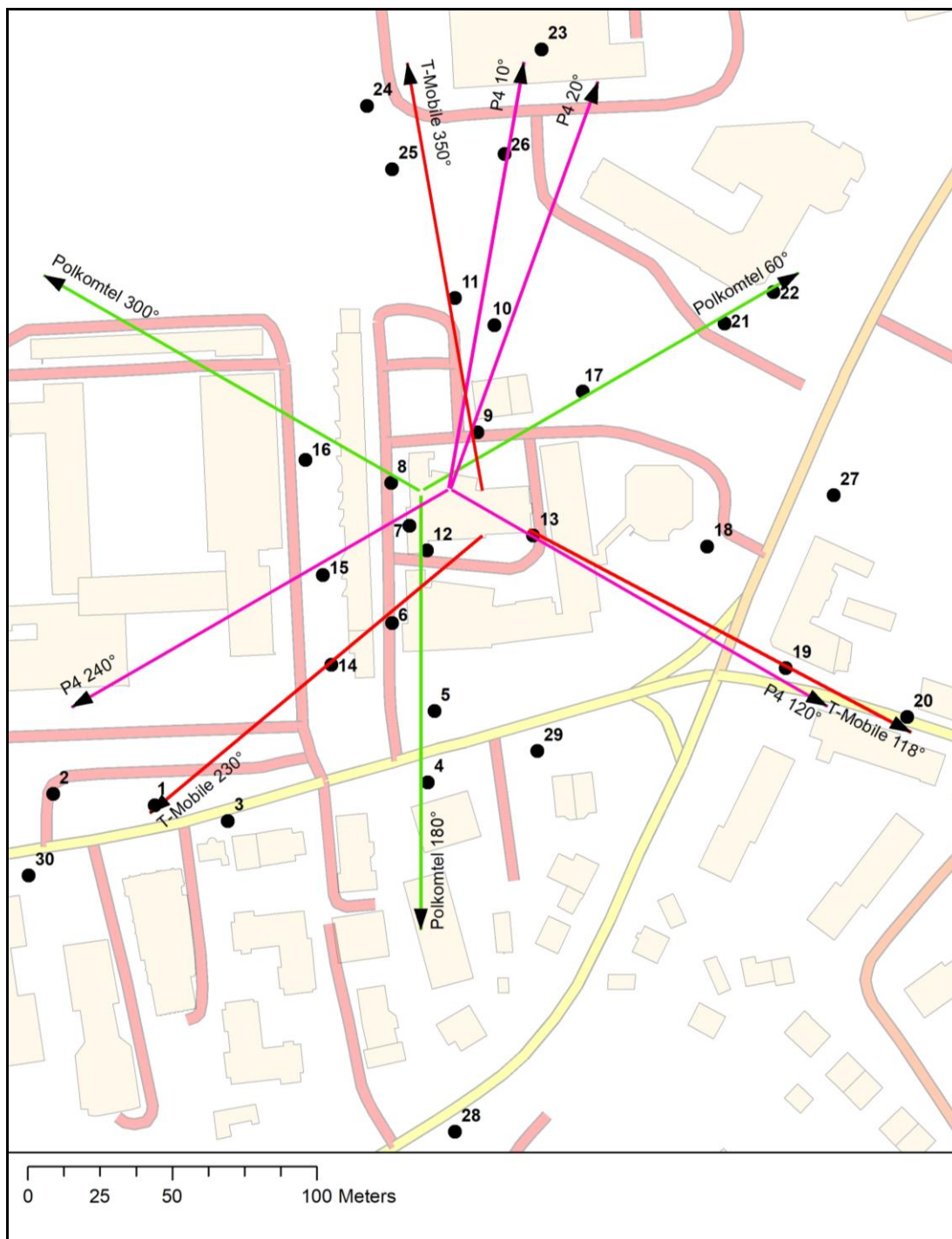
Rys. 1: Plan terenu, na którym znajdują się badane stacje bazowe
