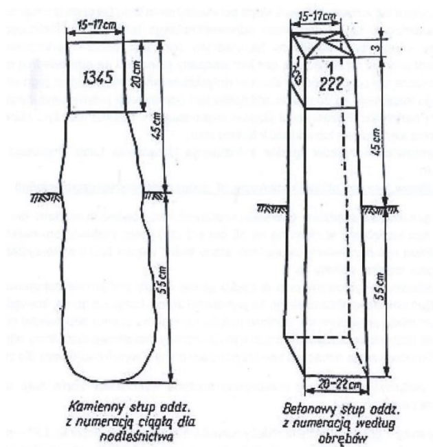
Rysunek 1. Parametry słupka kamiennego i betonowego wraz z oznaczeniem słupa oddziałowego.
