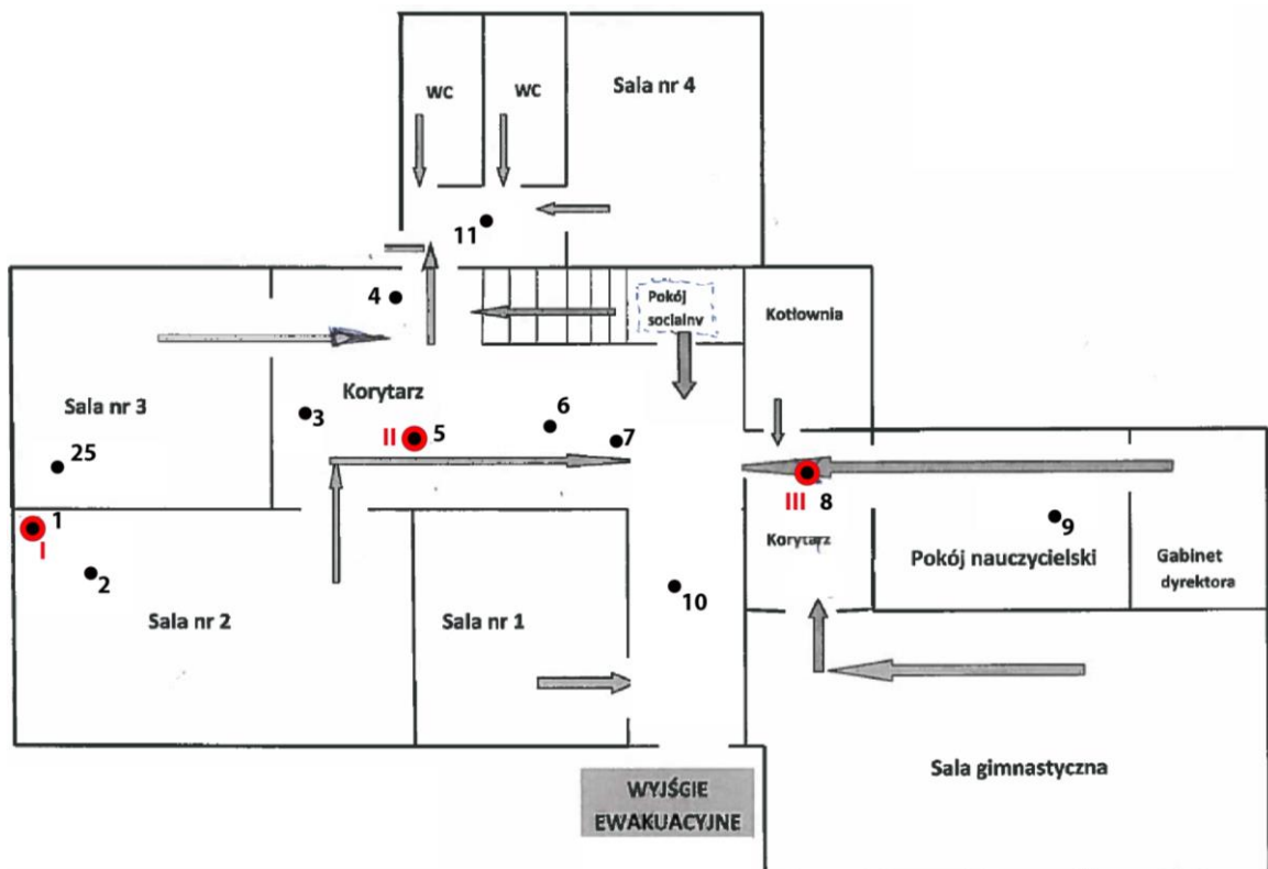
Rys. 1a: Plan rozmieszczenia punktów pomiarowych – parter kolorem czerwonym oznaczono lokalizację punktów dostępowych
