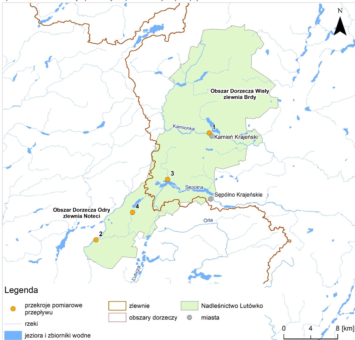
Rysunek 10. Lokalizacja przekrojów pomiarowych przepływu wód
