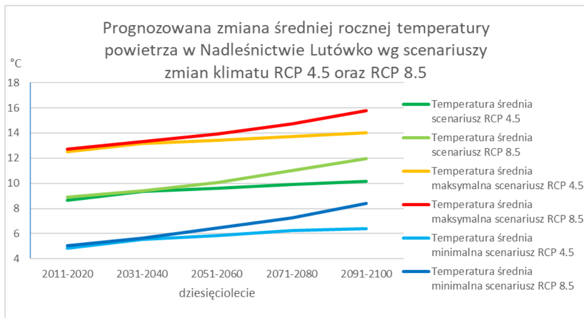
Rysunek 9 Prognozowana zmiana średniej rocznej, maksymalnej i minimalnej temperatury powietrza w Nadleśnictwie Lutówko w horyzoncie czasowym do 2100 roku wg scenariuszy zmian klimatu RCP 4.5 oraz RCP 8.5
