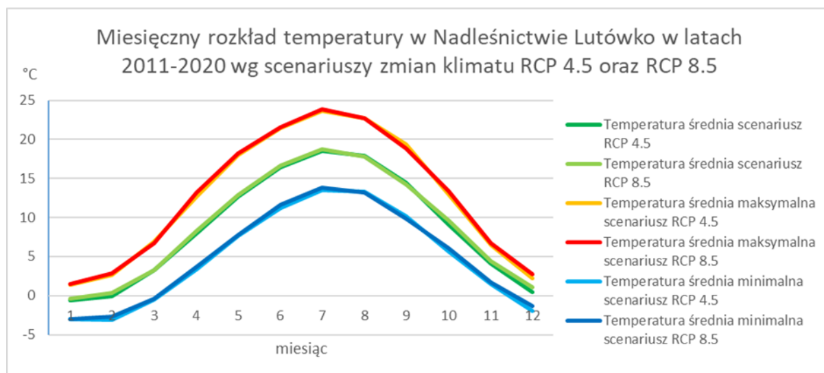
Rysunek 8 Miesięczny rozkład średniej, maksymalnej oraz minimalnej temperatury powietrza w Nadleśnictwie Lutówko w latach 2011-2020 wg scenariuszy zmian klimatu RCP 4.5 oraz RCP 8.5
