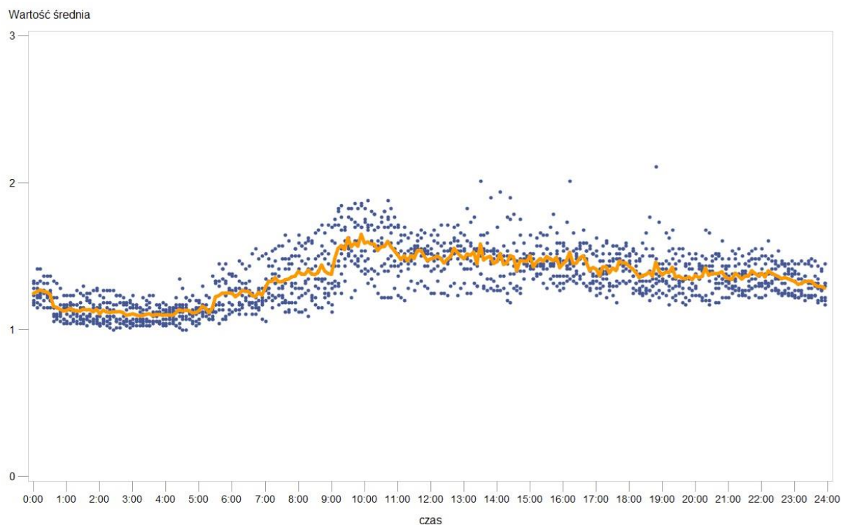
Rys. 7 Wyniki pomiarów – Zespół Sportowych Szkół Ogólnokształcących – średnia za okres 24 godzin
