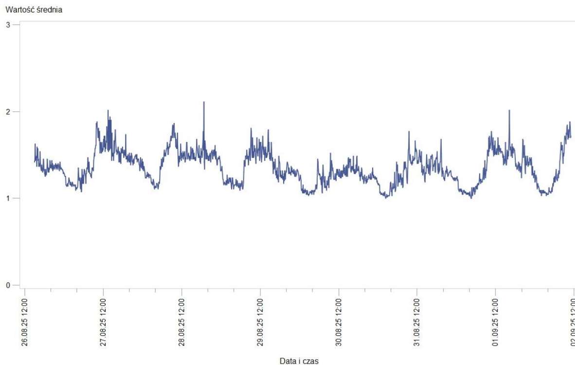
Rys. 5 Wyniki pomiarów – Zespół Sportowych Szkół Ogólnokształcących w dniach 26.08.2025 r. – 2.09.2025 r. – wartość średnia
