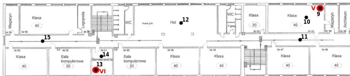
Rys. 1c: Plan rozmieszczenia punktów pomiarowych – II piętro, kolorem czerwonym oznaczono lokalizacje punktów dostępowych
