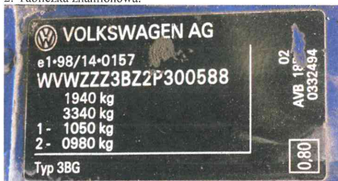
2. Tabliczka znamionowa.
