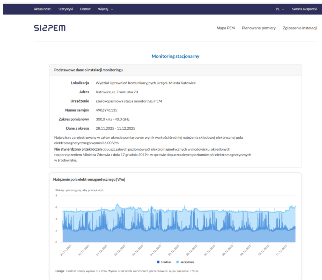
Rys. 23 Obrazowanie wyników monitoringu stacyjnego PEM – okres II
