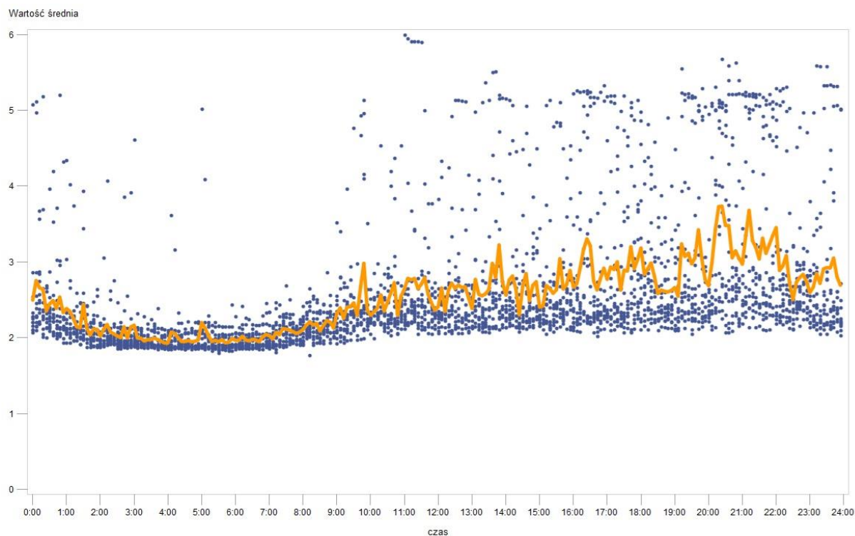
Rys. 11 Wyniki pomiarów – Urząd Miasta Katowice – średnia za okres 24 godzin – okres II
