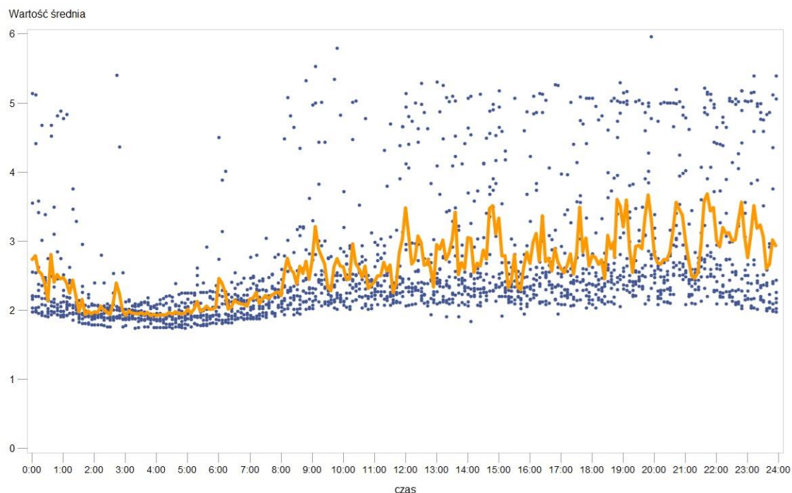
Rys. 8 Wyniki pomiarów – Urząd Miasta Katowice – średnia za okres 24 godzin -okres I
