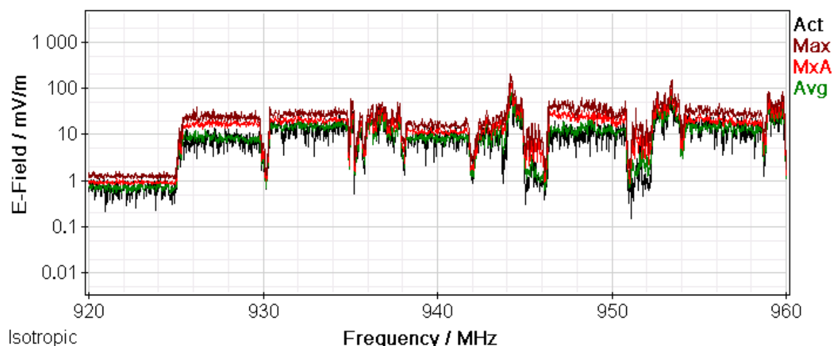
Rys. 15 Wyniki pomiarów selektywnych – zakres częstotliwości: 921,1 MHz – 959,9 MHz
