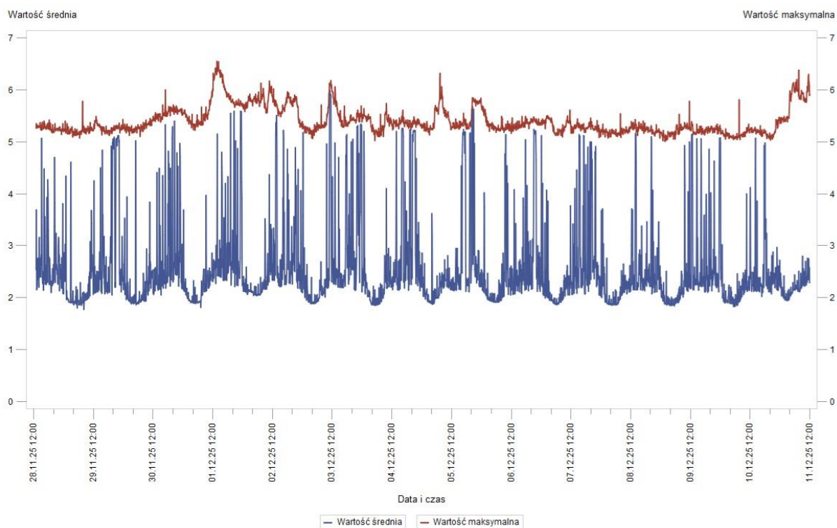
Rys. 10 Wyniki pomiarów – Urząd Miasta Katowice w dniach 28.11.2025 r. – 11.12.2025 r. – wartość średnia i wartość maksymalna
