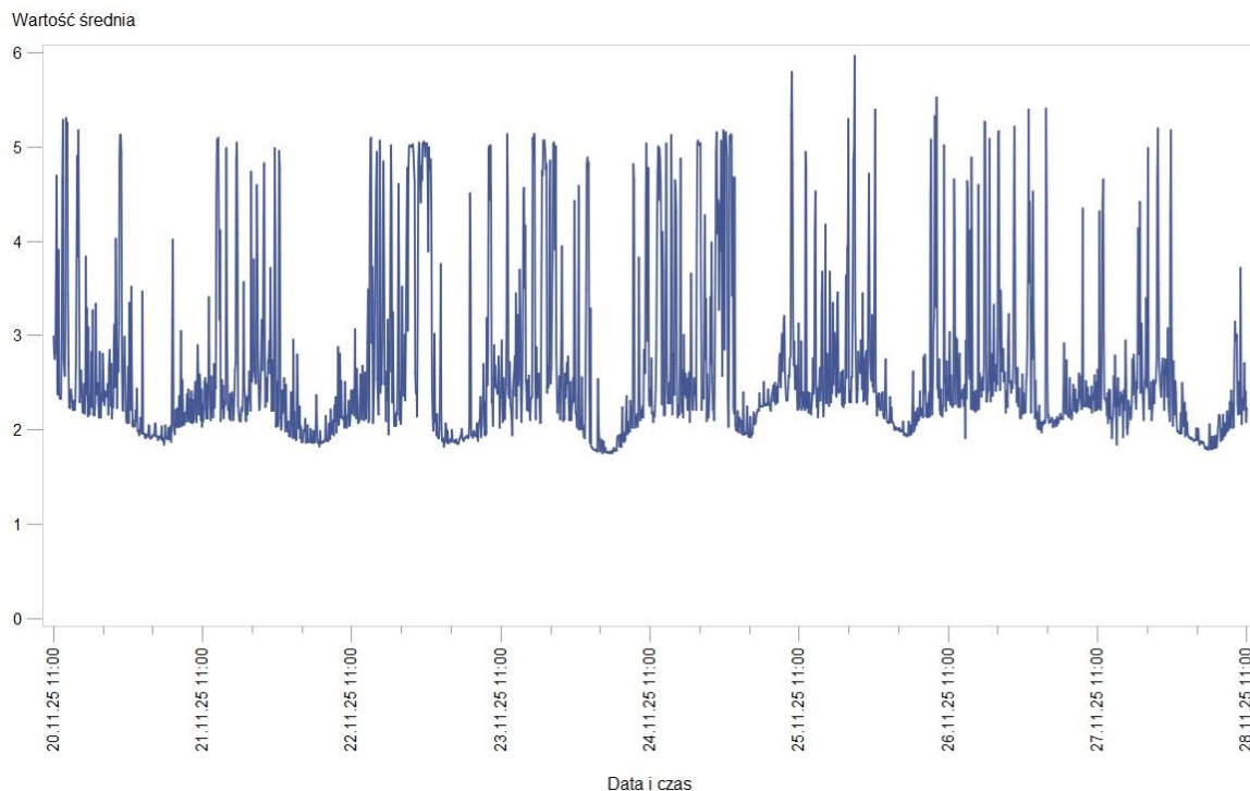
Rys. 6 Wyniki pomiarów – Urząd Miasta Katowice w dniach 20.11.2025 r. – 28.11.2025 r. – wartość średnia
