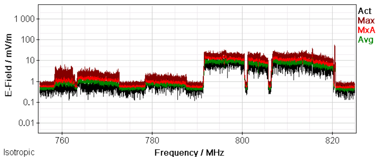
Rys. 14 Wyniki pomiarów selektywnych – zakresy częstotliwości: 750,0 MHz – 791,0 MHz oraz 791,0 MHz – 821,0 MHz
