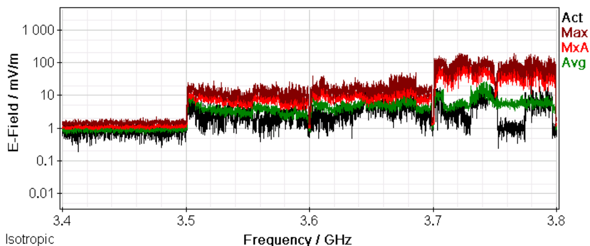
Rys. 19 Wyniki pomiarów selektywnych – zakres częstotliwości: 3400,0 MHz – 3800,0 MHz
