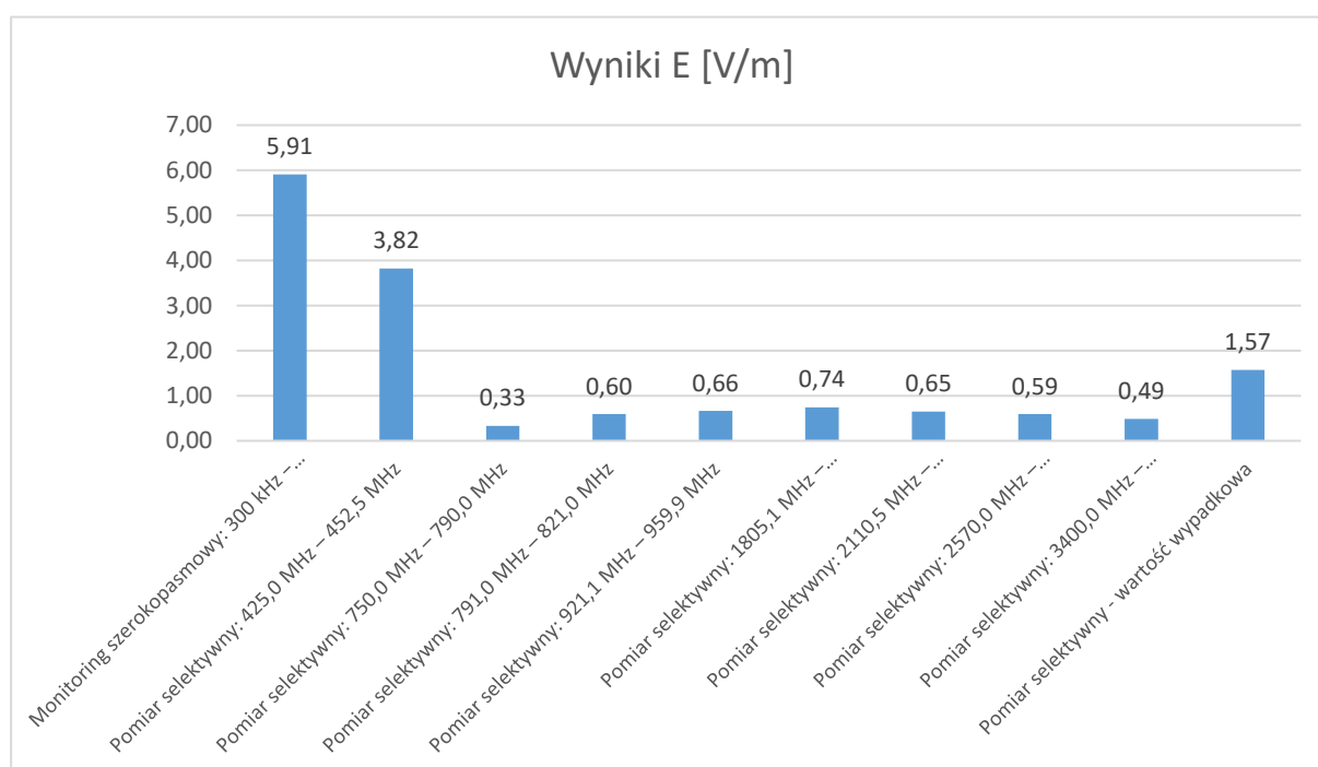
Rys. 20 Porównanie wyników monitoringu szerokopasmowego i pomiarów selektywnych
