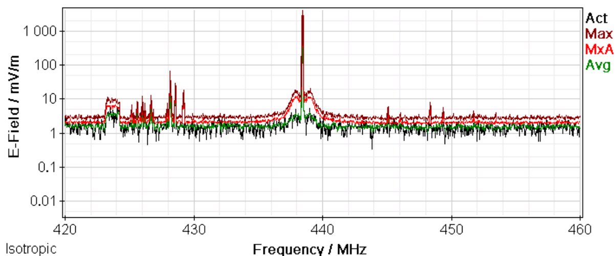
Rys. 13 Wyniki pomiarów selektywnych – zakres częstotliwości: 420,0 MHz – 460,0 MHz
