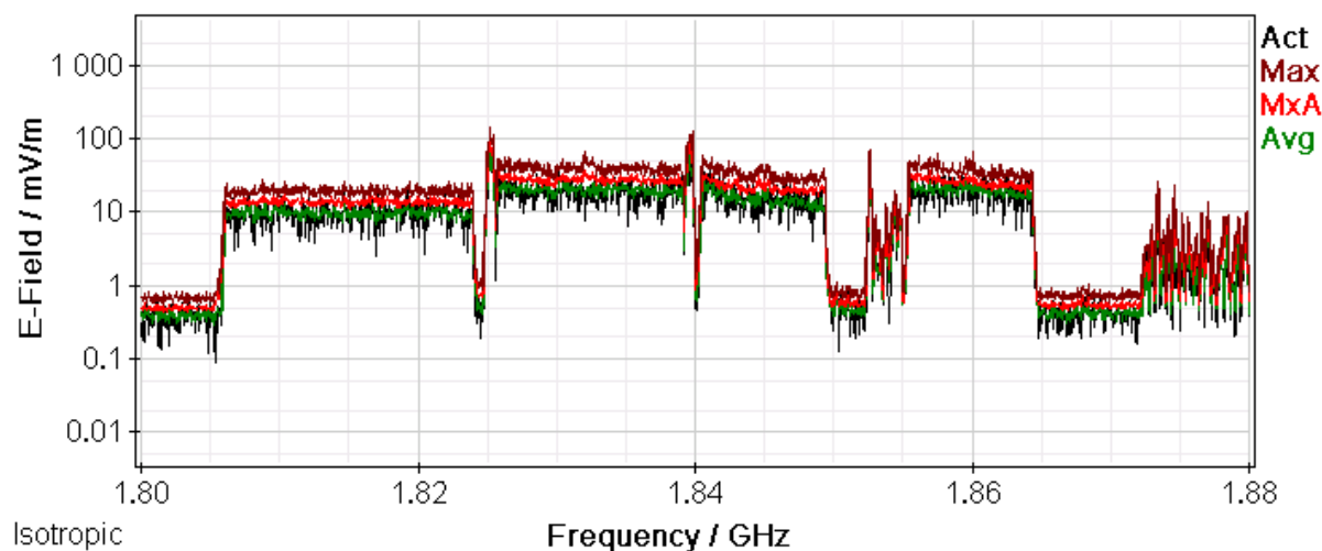
Rys. 16 Wyniki pomiarów selektywnych – zakres częstotliwości: 1805,1 MHz – 1879,9 MHz
