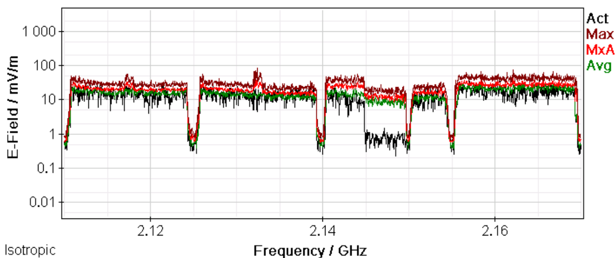
Rys. 17 Wyniki pomiarów selektywnych – zakres częstotliwości: 2110,5 MHz – 2169,7 MHz
