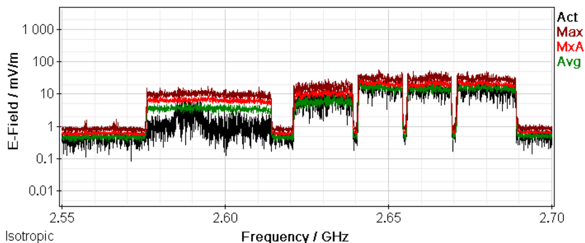
Rys. 18 Wyniki pomiarów selektywnych – zakres częstotliwości: 2570,0 MHz – 2690,0 MHz
