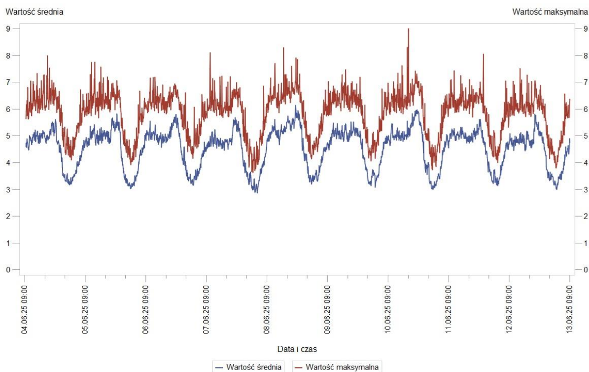
Rys. 6 Wyniki pomiarów – Budynek, ul. Batorego 34 w dniach 4.06.2025 r. – 13.06.2025 r. – wartość średnia i wartość maksymalna
