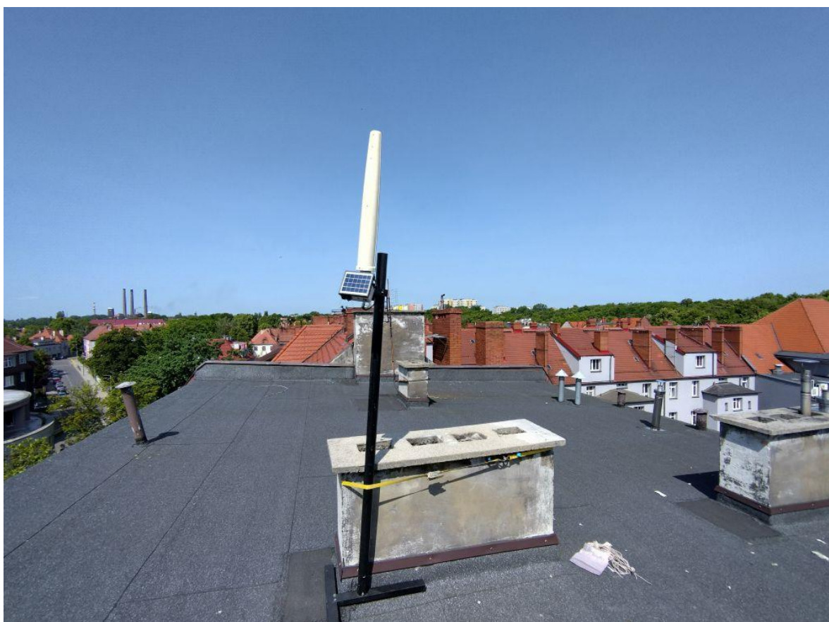
Rys. 2. Miejsce montażu SMS PEM – Budynek, ul. Batorego 34
