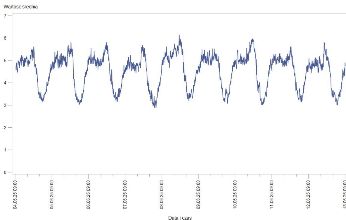
Rys. 5 Wyniki pomiarów – Budynek, ul. Batorego 34 w dniach 4.06.2025 r. – 13.06.2025 r. – wartość średnia
