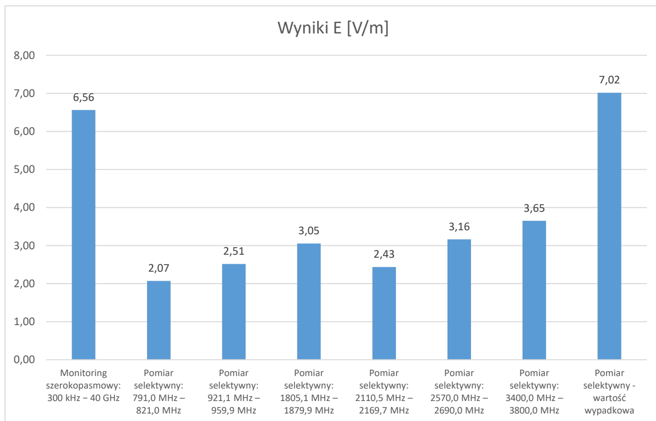
Rys. 15 Porównanie wyników monitoringu szerokopasmowego i pomiarów selektywnych
