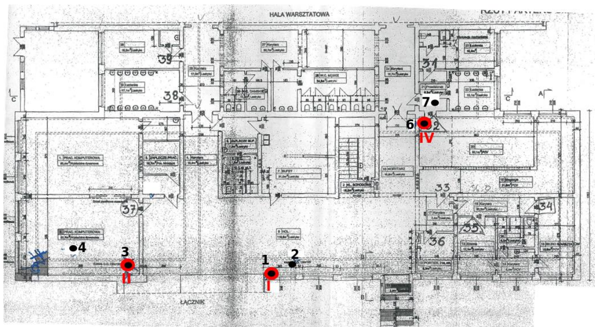
Rys. 1a: Plan rozmieszczenia punktów pomiarowych – parter, część administracyjna kolorem czerwonym oznaczono lokalizację punktów dostępowych
