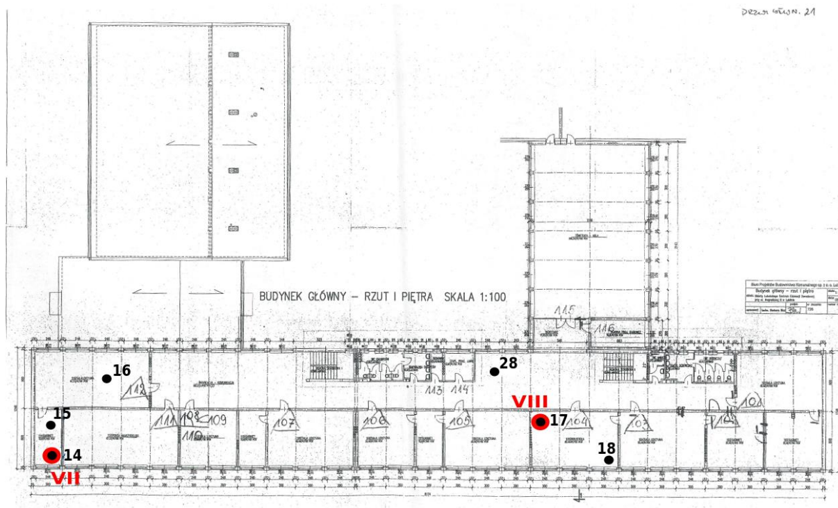
Rys. 1c: Plan rozmieszczenia punktów pomiarowych – I piętro, kolorem czerwonym oznaczono lokalizacje punktów dostępowych
