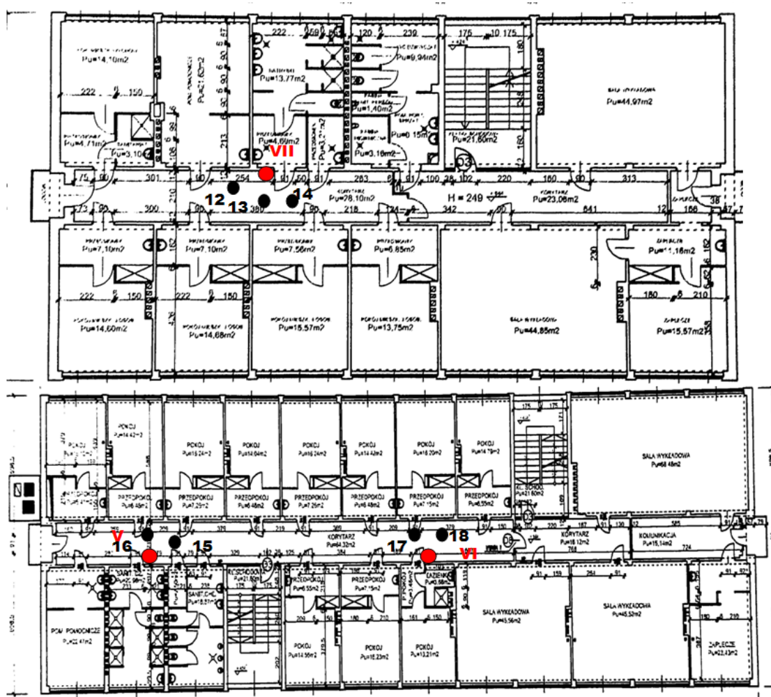
Rys. 1c: Plan rozmieszczenia punktów pomiarowych – II piętro, kolorem czerwonym oznaczono lokalizację punktów dostępowych
