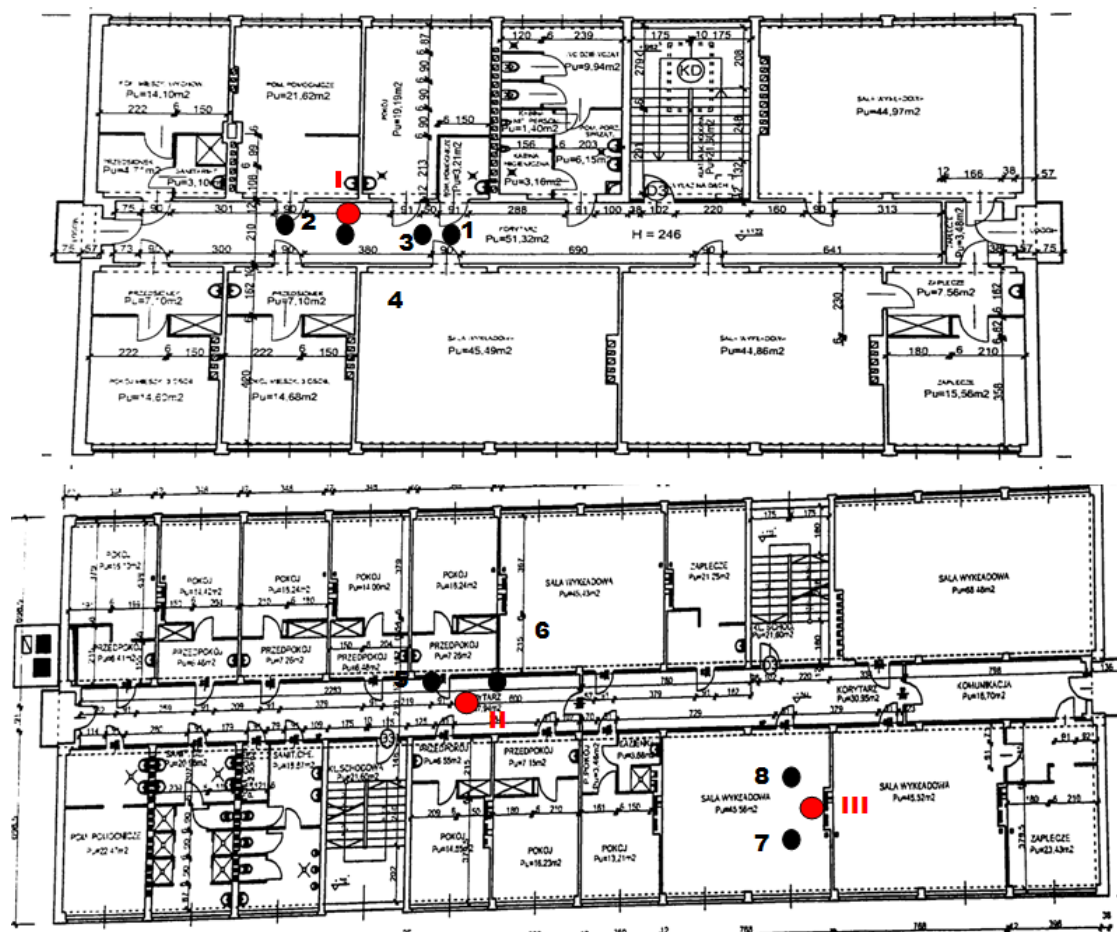
Rys. 1e: Plan rozmieszczenia punktów pomiarowych – IV piętro, kolorem czerwonym oznaczono lokalizację punktów dostępowych
