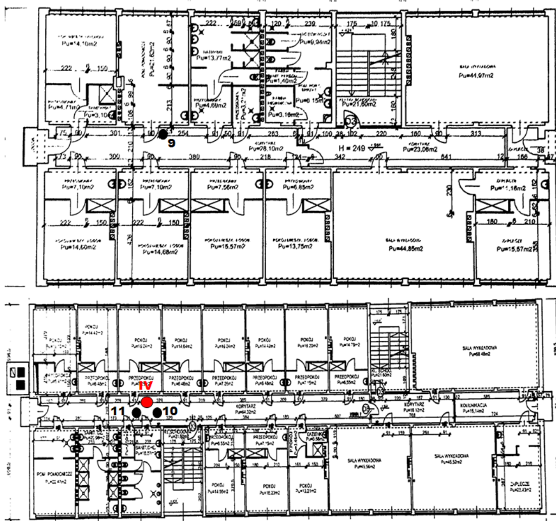
Rys. 1d: Plan rozmieszczenia punktów pomiarowych – III piętro, kolorem czerwonym oznaczono lokalizację punktów dostępowych
