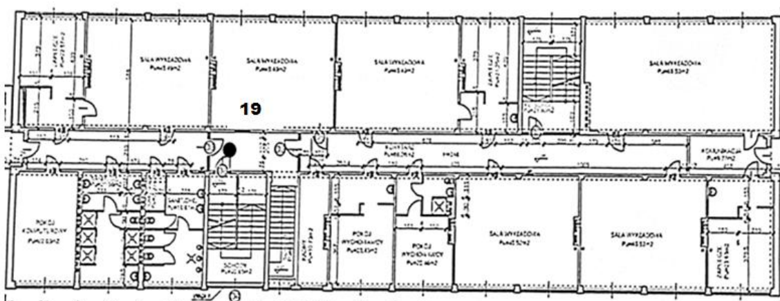
Rys. 1b: Plan rozmieszczenia punktów pomiarowych – I piętro
