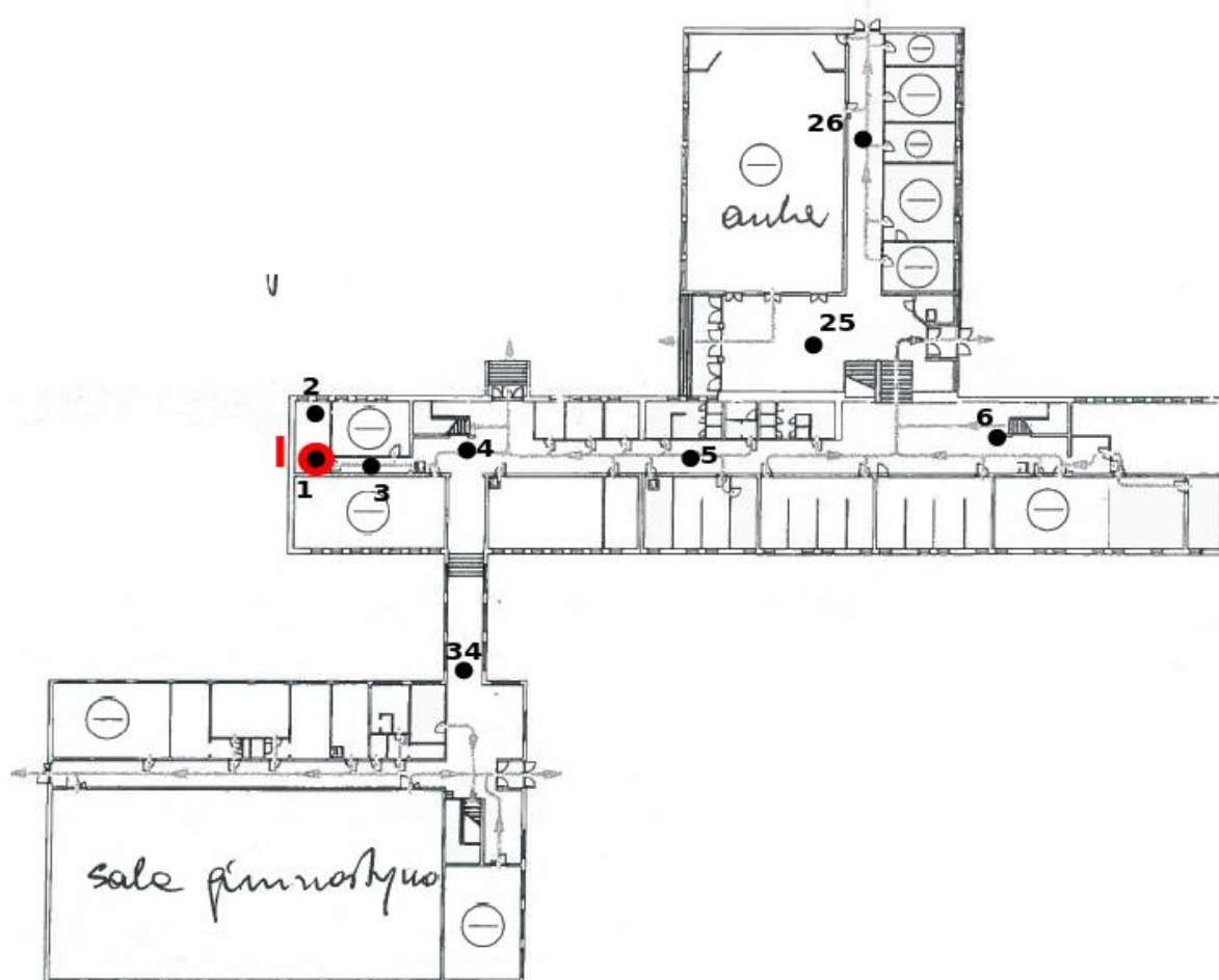
Rys. 1a: Plan rozmieszczenia punktów pomiarowych – piwnica i przyziemie, kolorem czerwonym oznaczono lokalizację punktów dostępowych
