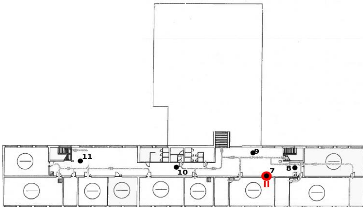
Rys. 1b: Plan rozmieszczenia punktów pomiarowych – parter, kolorem czerwonym oznaczono lokalizację punktu dostępowego
