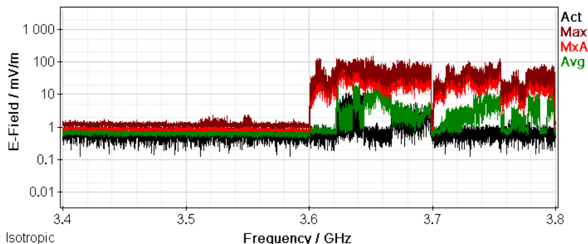
Rys. 15 Wyniki pomiarów selektywnych – zakres częstotliwości: 3400,0 MHz – 3800,0 MHz
