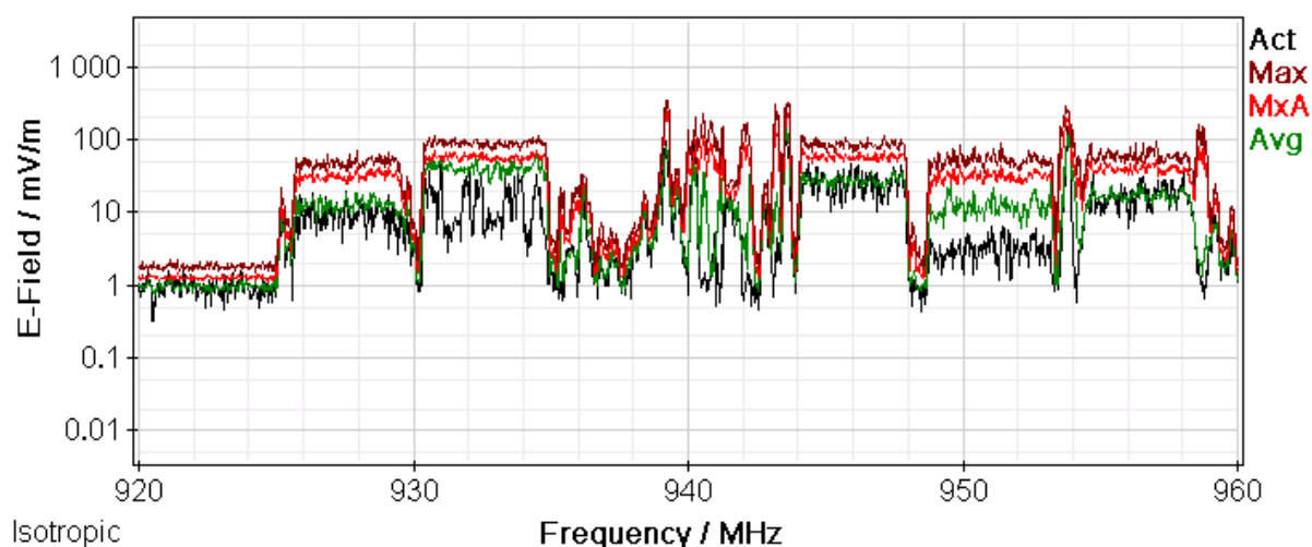
Rys. 11 Wyniki pomiarów selektywnych – zakres częstotliwości: 921,1 MHz – 959,9 MHz
