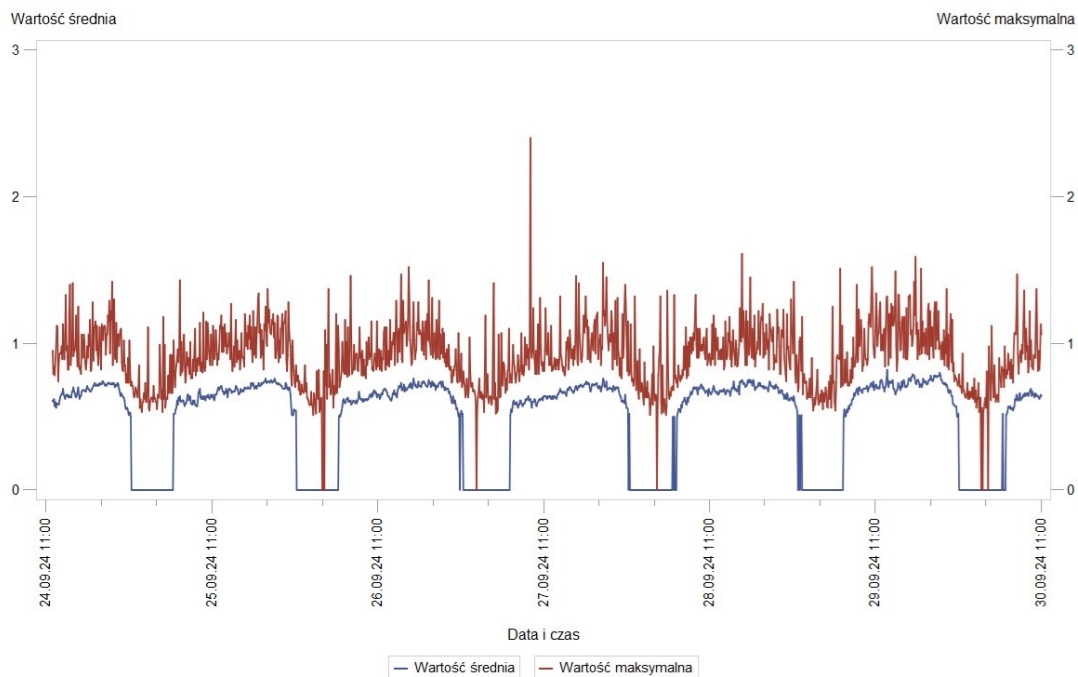
Rys. 7 Wyniki pomiarów – DPS w Suwałkach w dniach 24.09.2024 r. – 30.09.2024 r. – wartość średnia i wartość maksymalna
