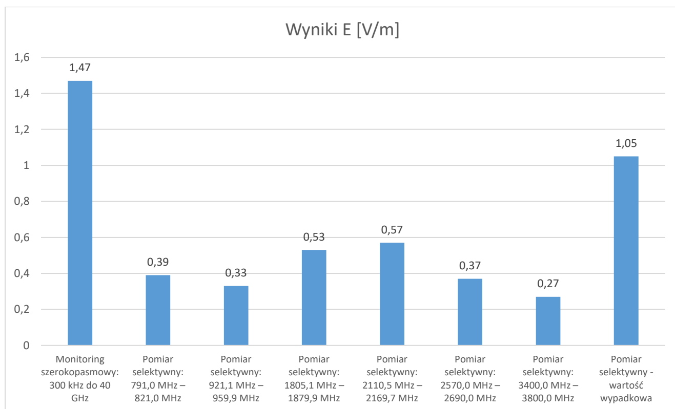
Rys. 16 Porównanie wyników monitoringu szerokopasmowego i pomiarów selektywnych
