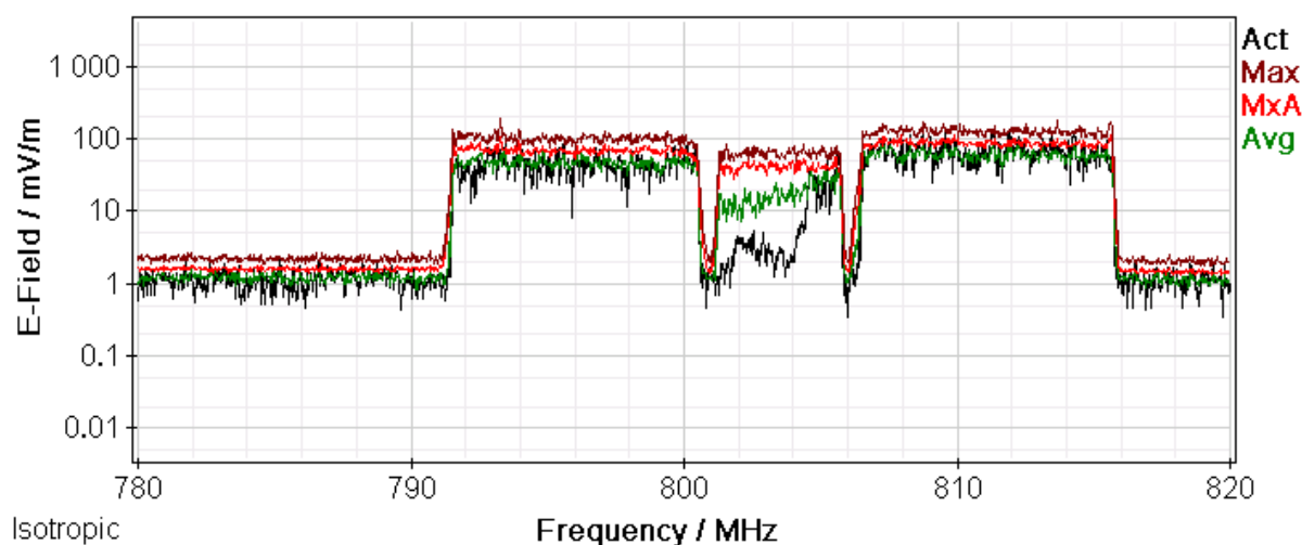
Rys. 10 Wyniki pomiarów selektywnych – zakres częstotliwości: 791,0 MHz – 821,0 MHz
