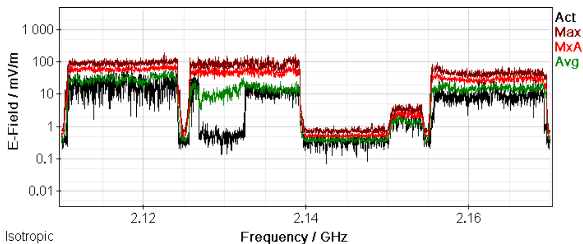
Rys. 13 Wyniki pomiarów selektywnych – zakres częstotliwości: 2110,5 MHz – 2169,7 MHz
