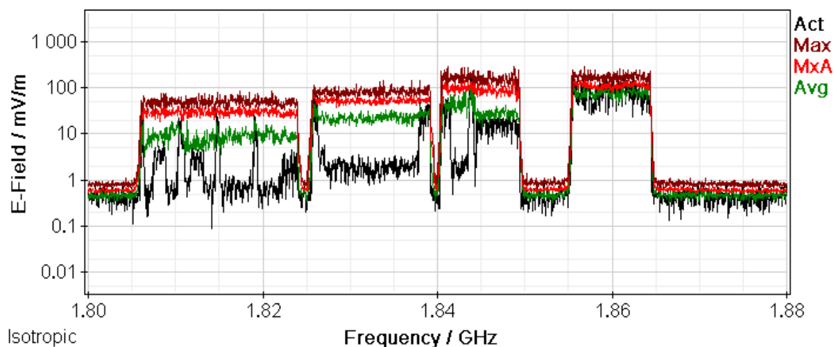
Rys. 12 Wyniki pomiarów selektywnych – zakres częstotliwości: 1805,1 MHz – 1879,9 MHz
