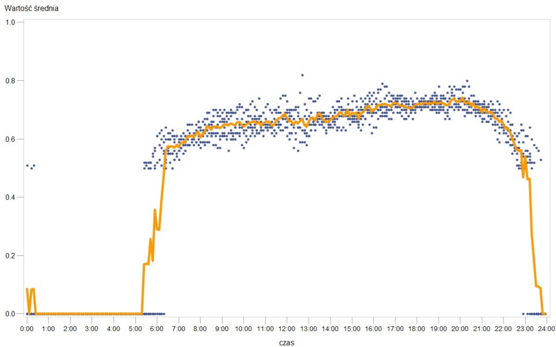
Rys. 8 Wyniki pomiarów – DPS w Suwałkach – średnia za okres 24 godzin
