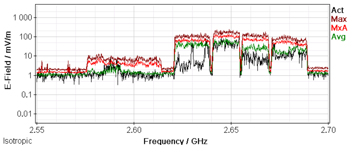
Rys. 14 Wyniki pomiarów selektywnych – zakres częstotliwości: 2570,0 MHz – 2690,0 MHz
