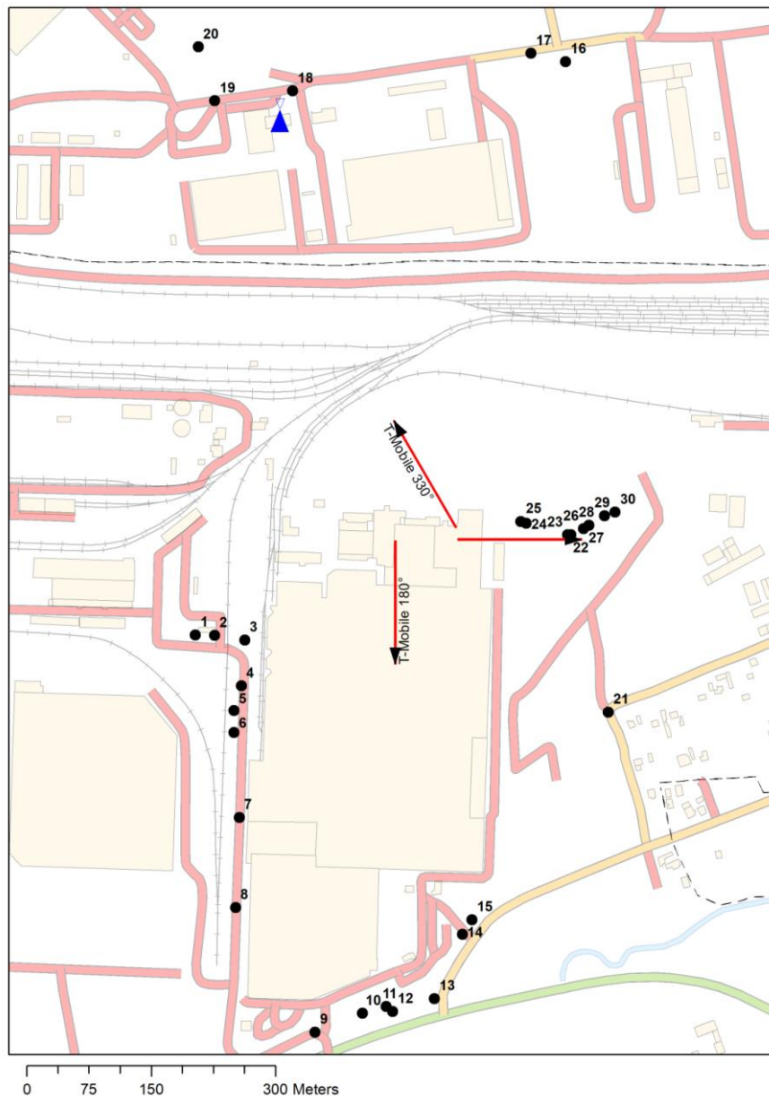
Rys. 1: Plan terenu, na którym znajduje się badana stacja bazowa
