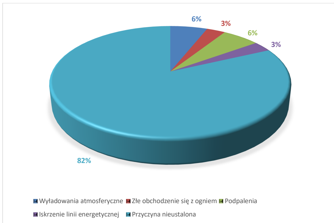
Ryc. 21 Przyczyny pożarów
