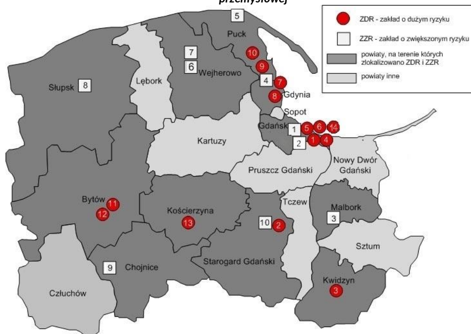
Rysunek 18. Lokalizacja zakładów dużego i zwiększonego ryzyka wystąpienia poważnej awarii przemysłowej
