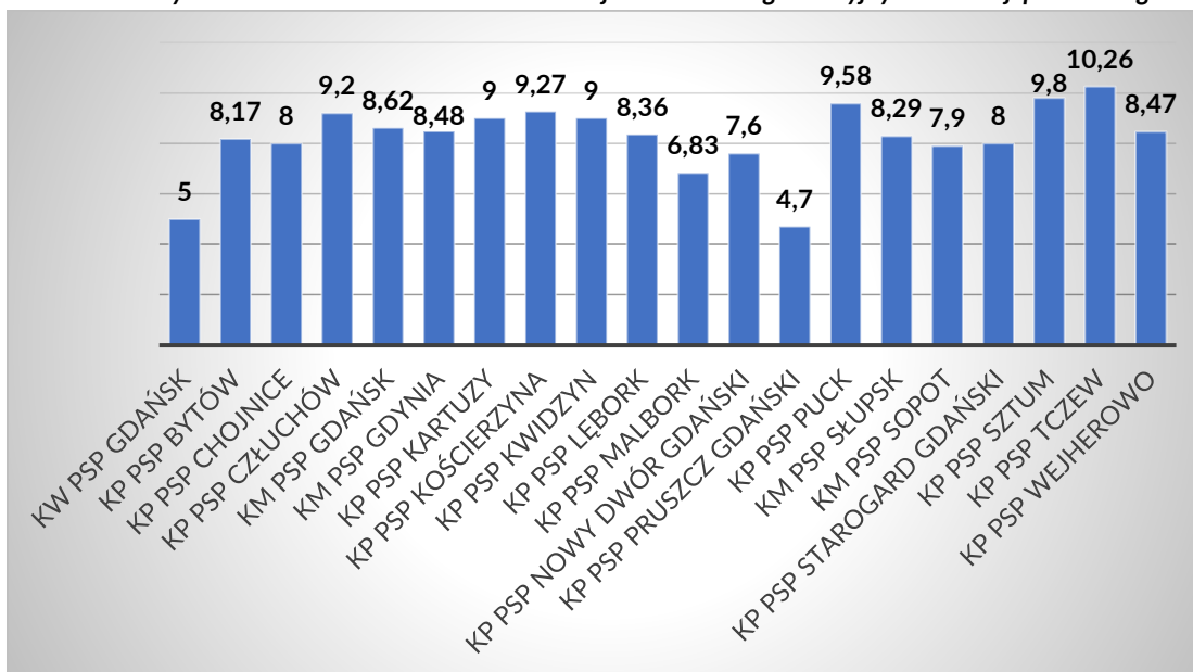
Rysunek 20. Średni wiek samochodów w jednostkach organizacyjnych PSP woj. pomorskiego
