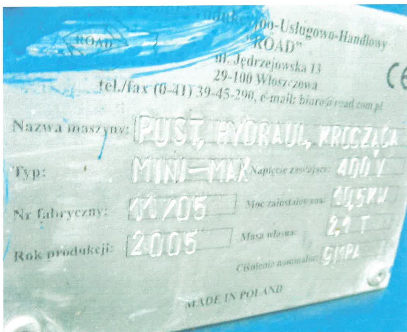
PUSTACZARKA HYDRAULICZNA KROCZĄCA MINI-MAX ROK PRODUKCJI 2005
