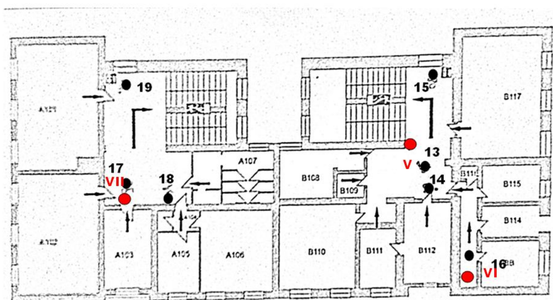
Rys. 1b: Plan rozmieszczenia punktów pomiarowych – I piętro, kolorem czerwonym oznaczono lokalizację punktów dostępnych
