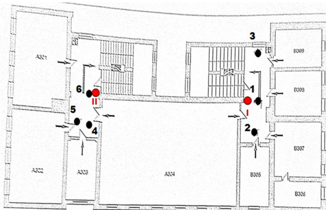
Rys. 1d: Plan rozmieszczenia punktów pomiarowych – III piętro, kolorem czerwonym oznaczono lokalizację punktów dostępowych
