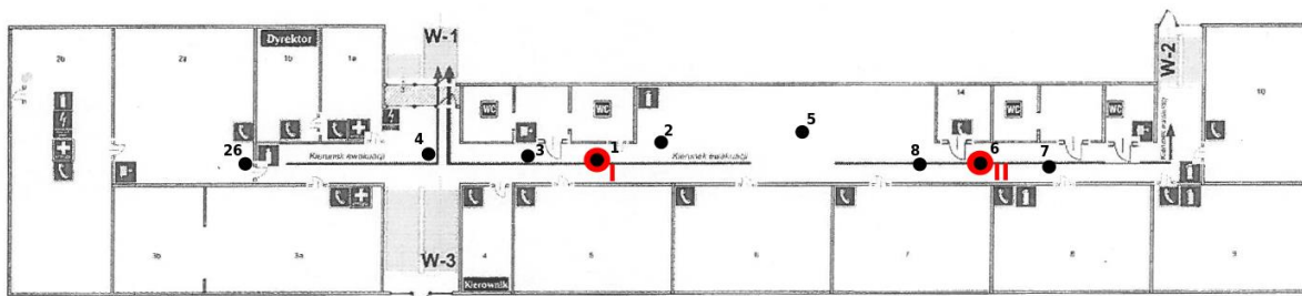
Rys. 1a: Plan rozmieszczenia punktów pomiarowych – parter, kolorem czerwonym oznaczono lokalizację punktów dostępowych
