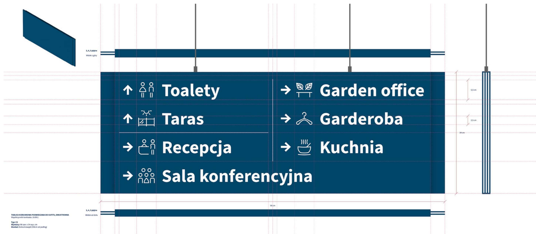
Rys. 3. Tablice podwieszane (C2)
