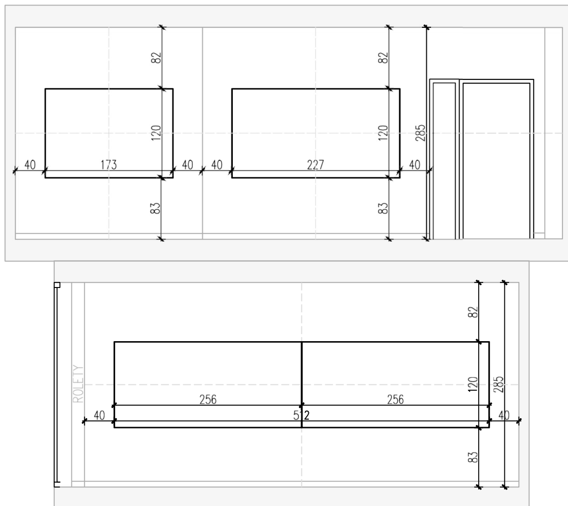
Rys. 16. Panele akustyczne w pomieszczeniu 5.012
