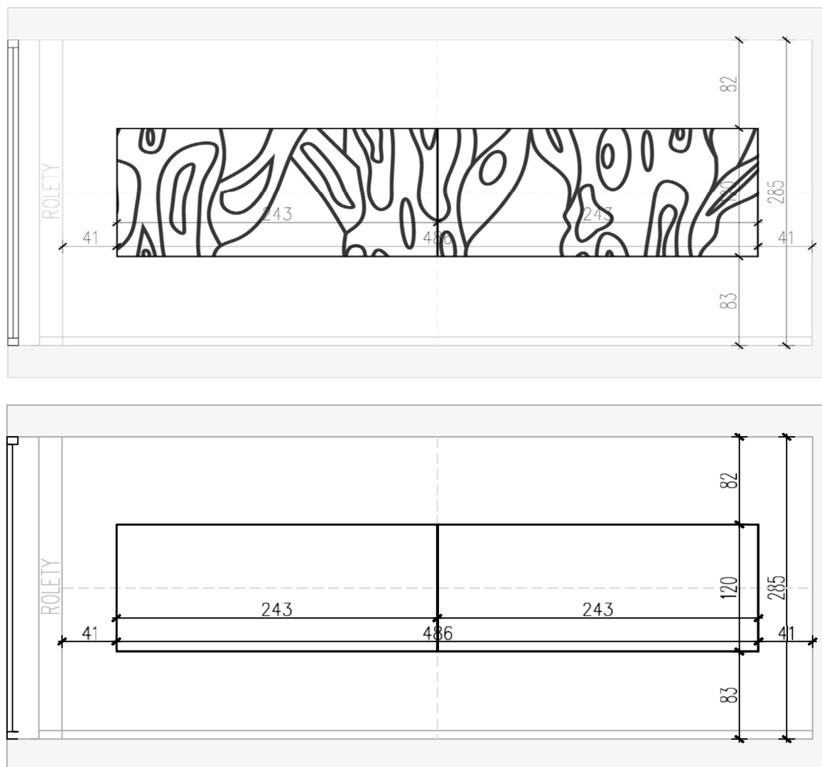
Rys. 14. Panel akustyczny w pomieszczeniu 5.049
