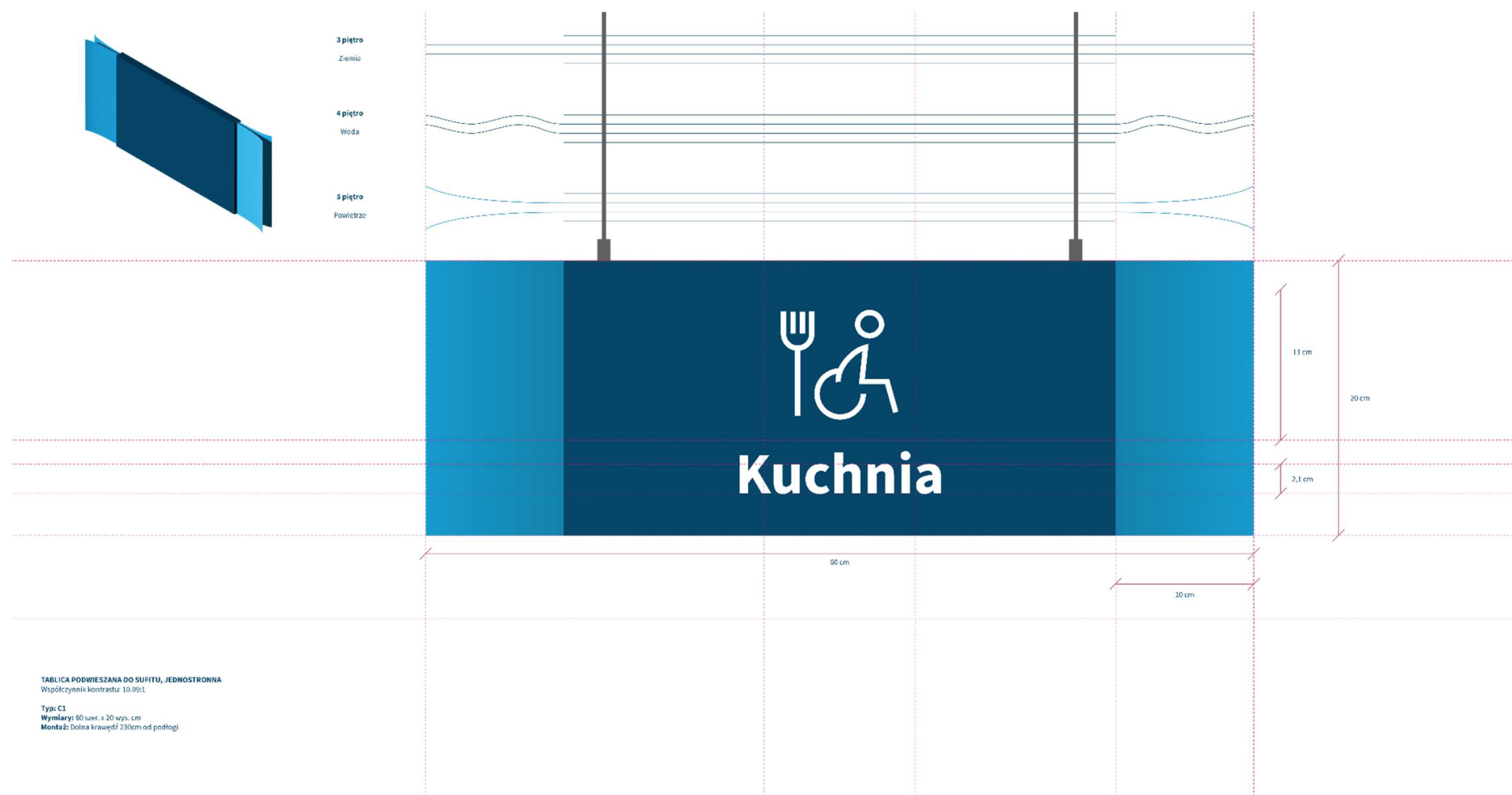
Rys. 2. Tablice podwieszane (C1)
