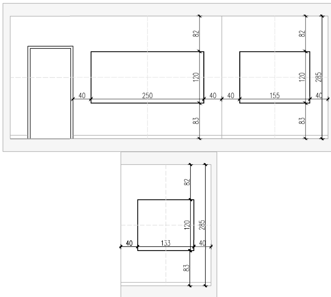
Rys. 15. Panele akustyczne w pomieszczeniu 5.001
