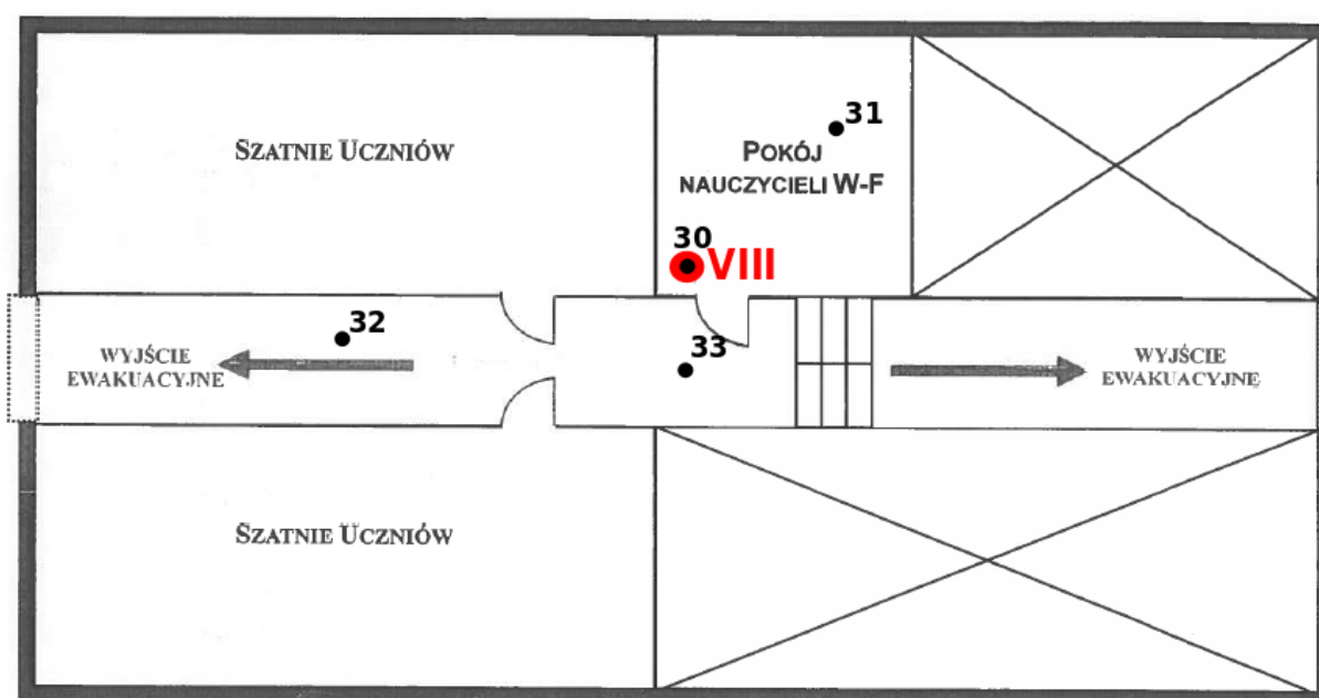
Rys. 1b: Plan rozmieszczenia punktów pomiarowych – parter, część B, kolorem czerwonym oznaczono lokalizację punktów dostępnych.
