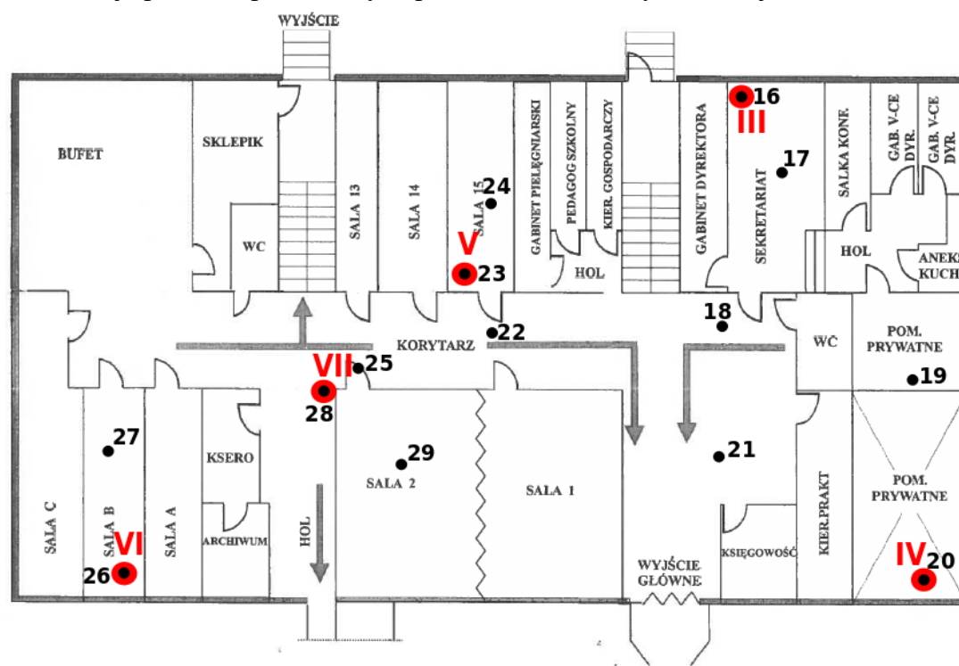
Rys. 1a: Plan rozmieszczenia punktów pomiarowych – parter, kolorem czerwonym oznaczono lokalizację punktów dostępnych.
