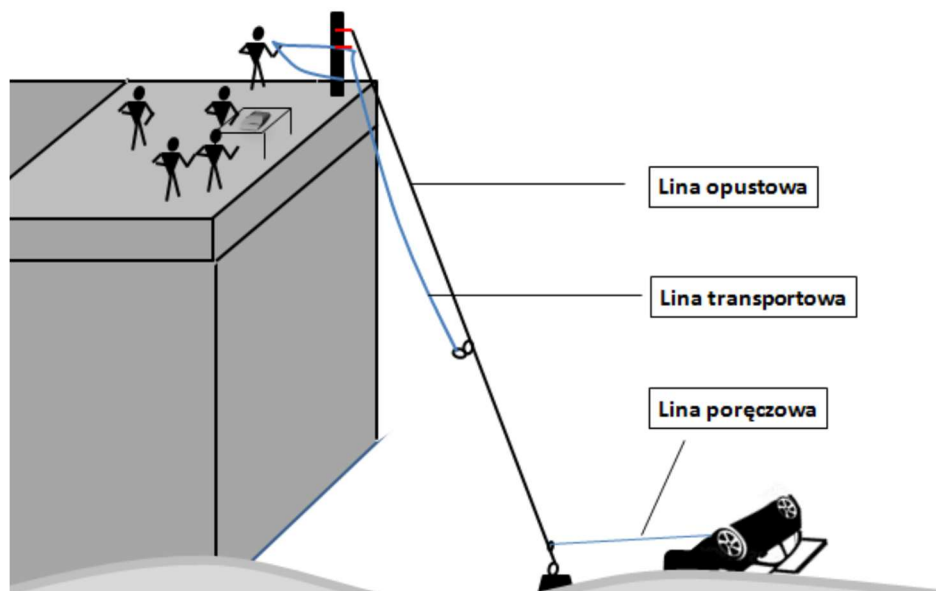
rys. 222 Metoda transportu sprzętu z bazy nurkowej do nurka
