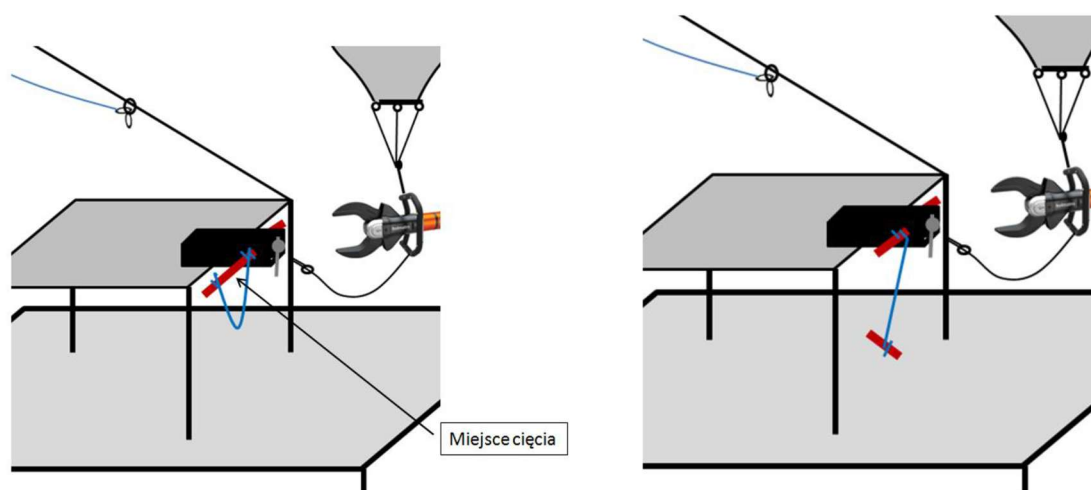
rys. 234 Zabezpieczenie przy pomocy linki elementu ciętego
