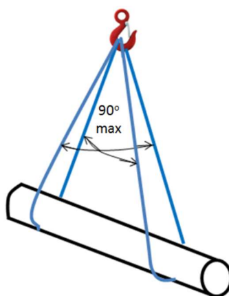
rys. 217 Instrukcja mocowania zawiesi
