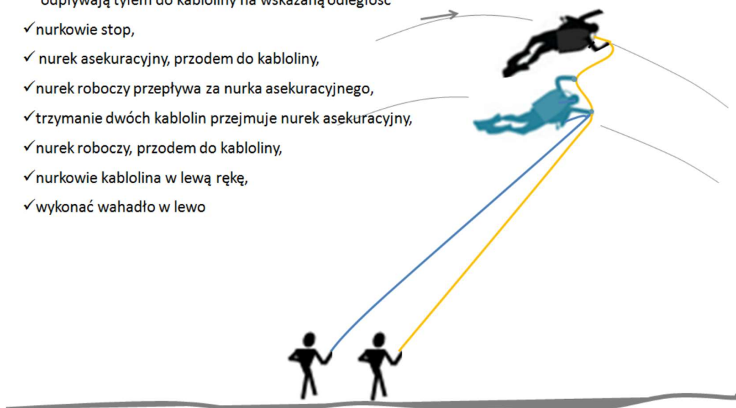
rys. 191 Poruszanie się na wahadle w parze nurkowej
