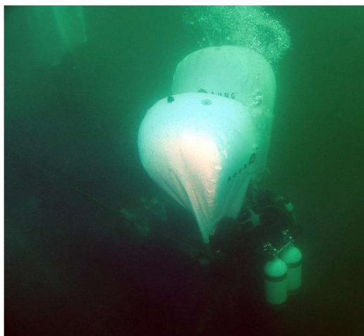
rys. 224 Wydobycie obiektu na powierzchnię wody z zastosowaniem balonów wypornościowych Fot. mł. bryg. Paweł Dyba, SGRW-N „Małopolska”
