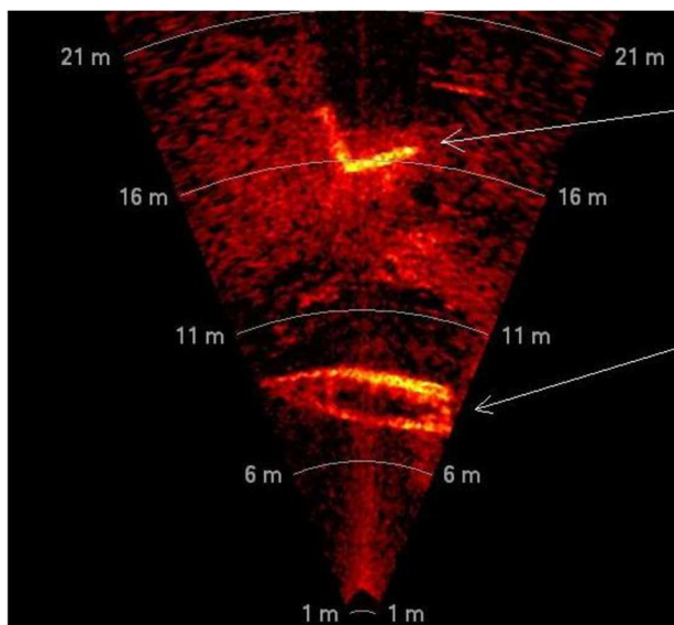
rys. 157 Obraz widziany z bezałogowego pojazdu podwodnego ROV Video Ray Pro 3XE GTO, wyposażonego w kamerę oraz w sonar czołowy.
