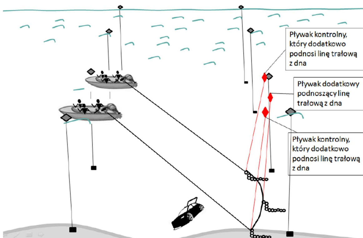
rys. 160 Trał denny (rys. powyżej) i trał o stałej głębokości zanurzenia (rys. poniżej)
