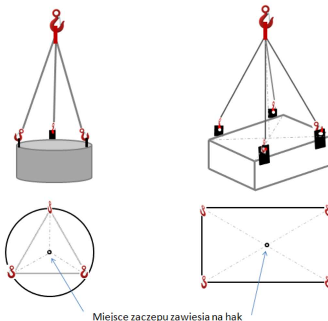
rys. 210 Symetryczne zawieszanie
