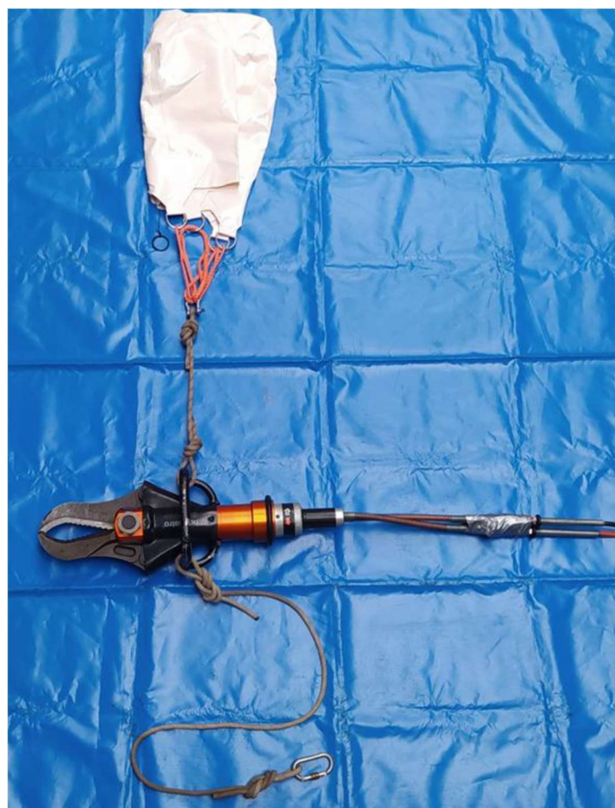
rys. 230 Odciężenie urządzenia technicznego stosowanego do cięcia hydraulicznego
