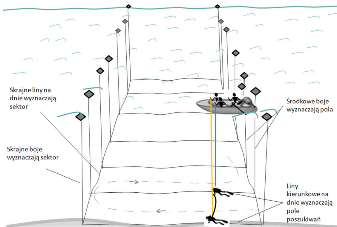
rys. 207 Metoda poszukiwań polami przez dwóch nurków z wykorzystaniem liny trałowej
