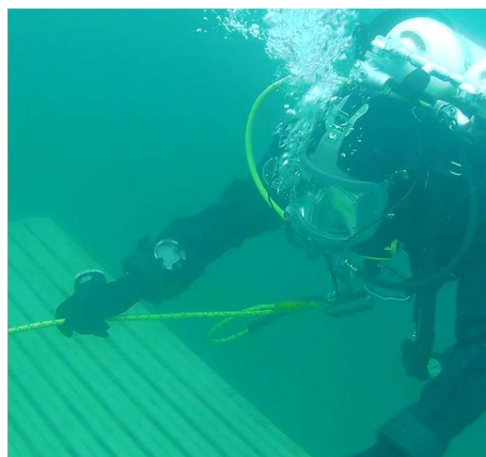
rys. 173 Instrukcja wykonania wahadła w prawo pod wodą
