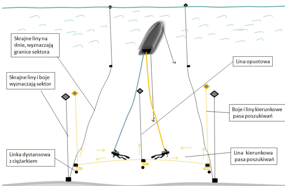
rys. 198 Metoda wahadłowa pasami dla dwóch nurków
