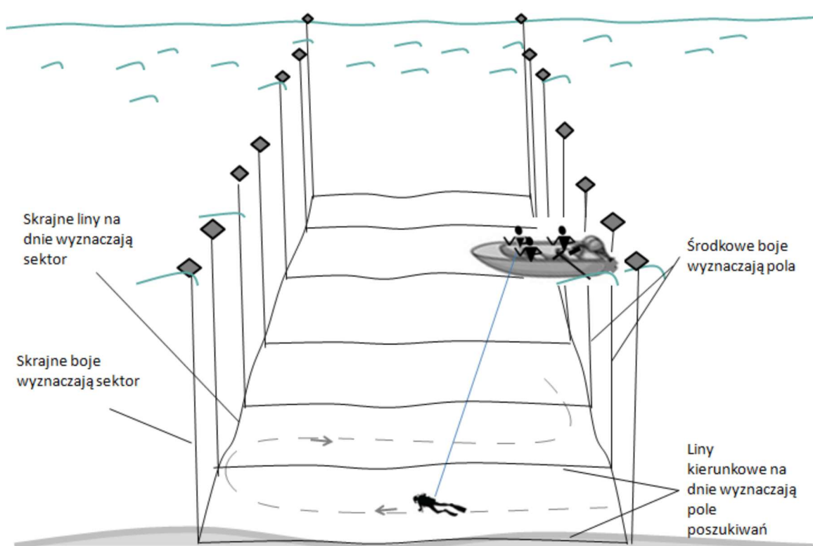
rys. 206 Metoda wyznaczonymi polami
