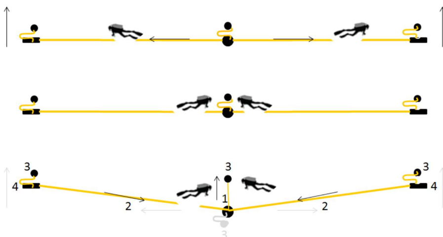
rys. 200 Sposób poruszania się w metodzie wahadłowej pasami przez dwóch nurków
