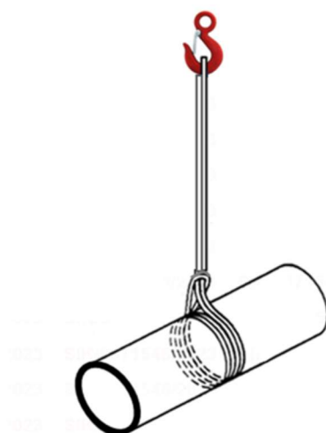
rys. 216 Instrukcja mocowania zawiesi
