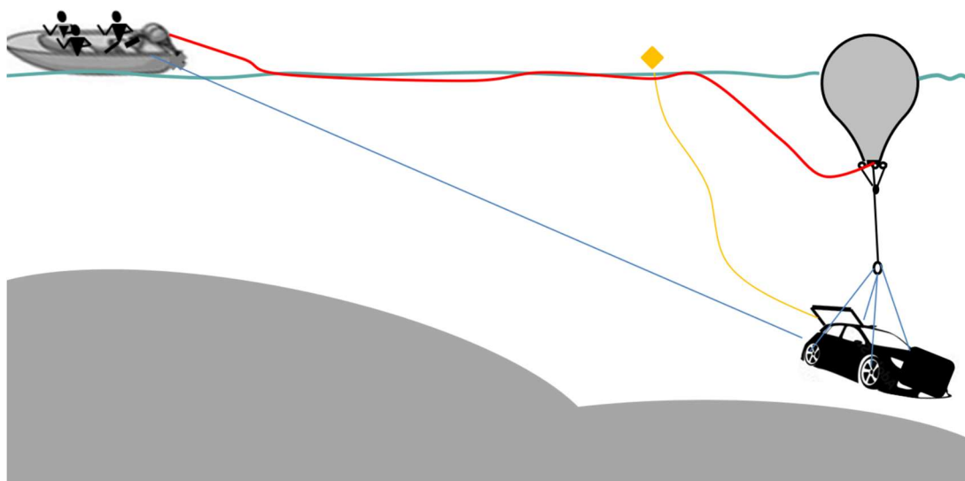
rys. 222 Wydobycie ciężkiego obiektu z większej głębokości z użyciem długiego zawiesia
