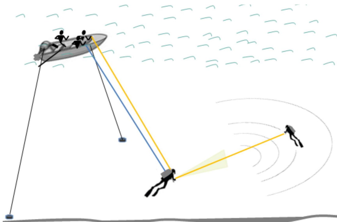
rys. 196 Metoda wahadłowa prowadzona przez dwóch nurków, gdzie nurek asekuracyjny wypuszcza nurka roboczego
