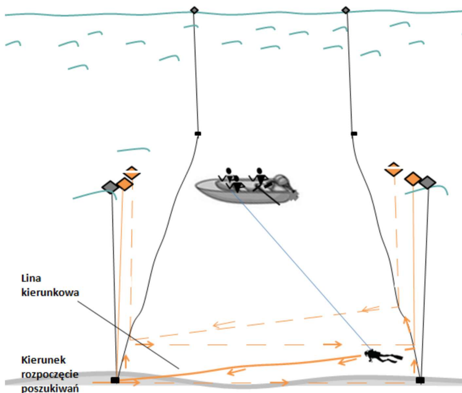
rys. 201 Metoda wahadłowa pasami dla jednego lub dwóch nurków
