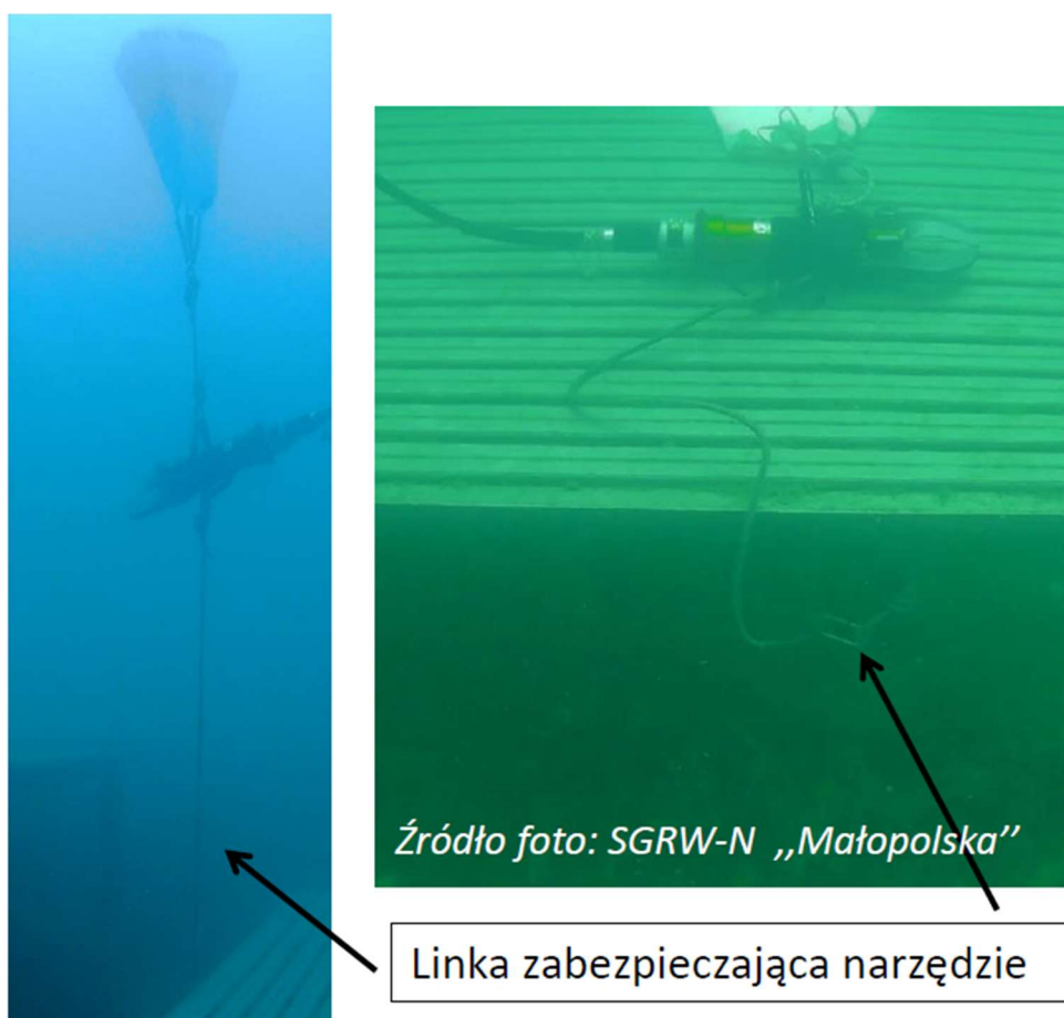
rys. 233 Odciążenie urządzenia technicznego stosowanego do cięcia hydraulicznego Fot. SGRW-N „Małopolska”
