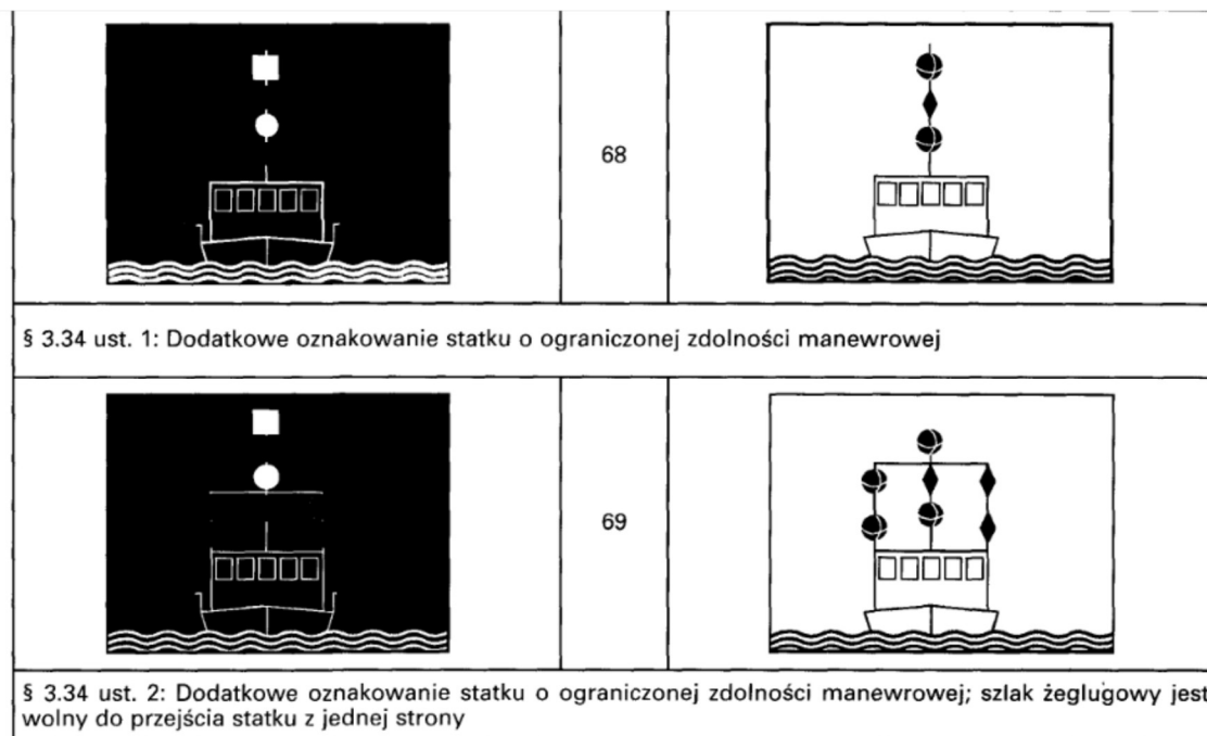
rys. 148 Dodatkowe oznakowanie statku o ograniczonej zdolności manewrowej
