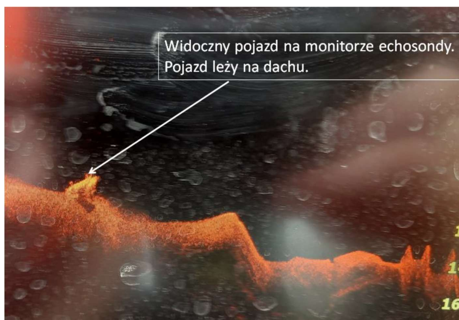
rys. 154 Obrazy z echosondy
