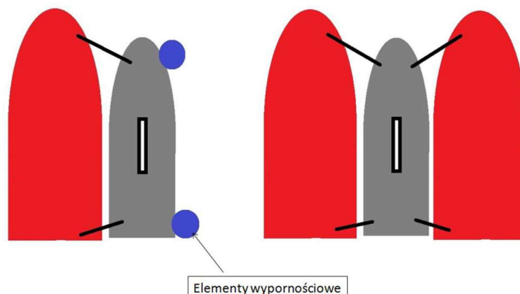
rys. 237 Instrukcja podłączenia lin do wywróconej jednostki Fot. Mazurskie Ochotnicze Pogotowie Ratunkowe Giżycko
