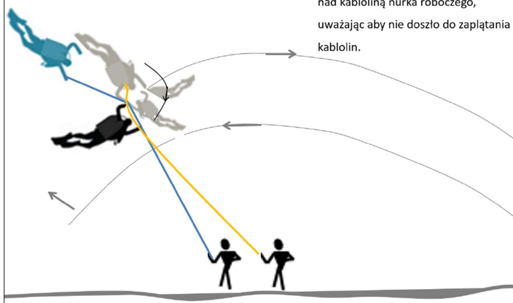
rys. 184 Poruszanie się na wahadle w parze nurkowej
