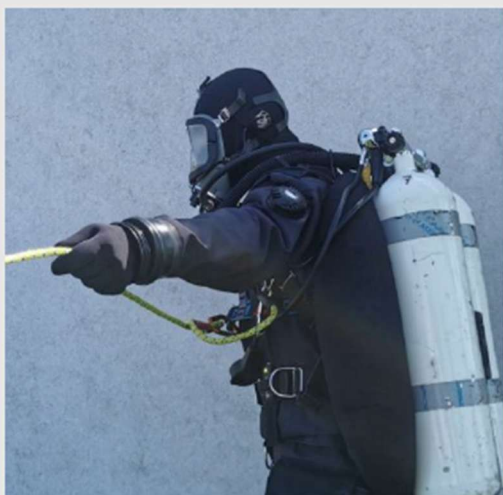
rys. 175 Instrukcja trzymania kabloliny w trakcie wahadła w lewo
