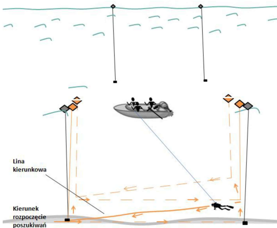
rys. 202 Uproszczona metoda wahadłowa pasami
