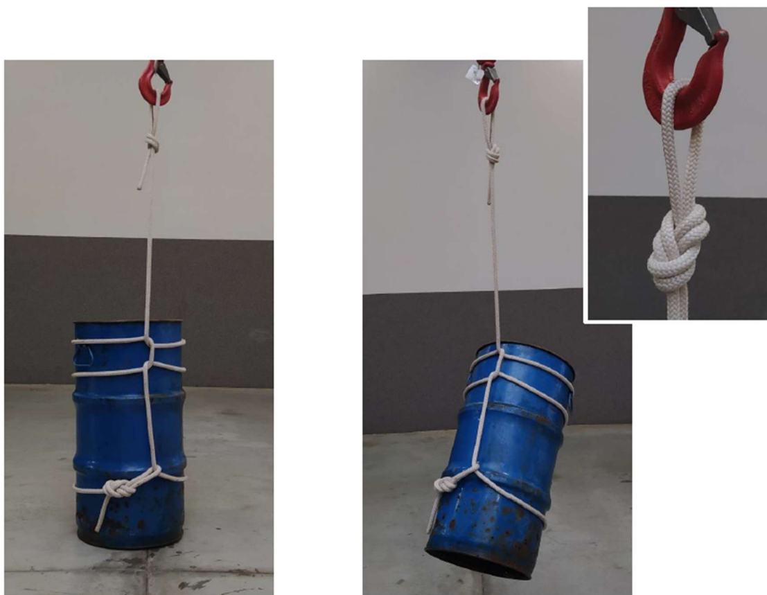
rys. 219 Prezentacja zastosowania zawiesi jedno- lub dwucięnowych
