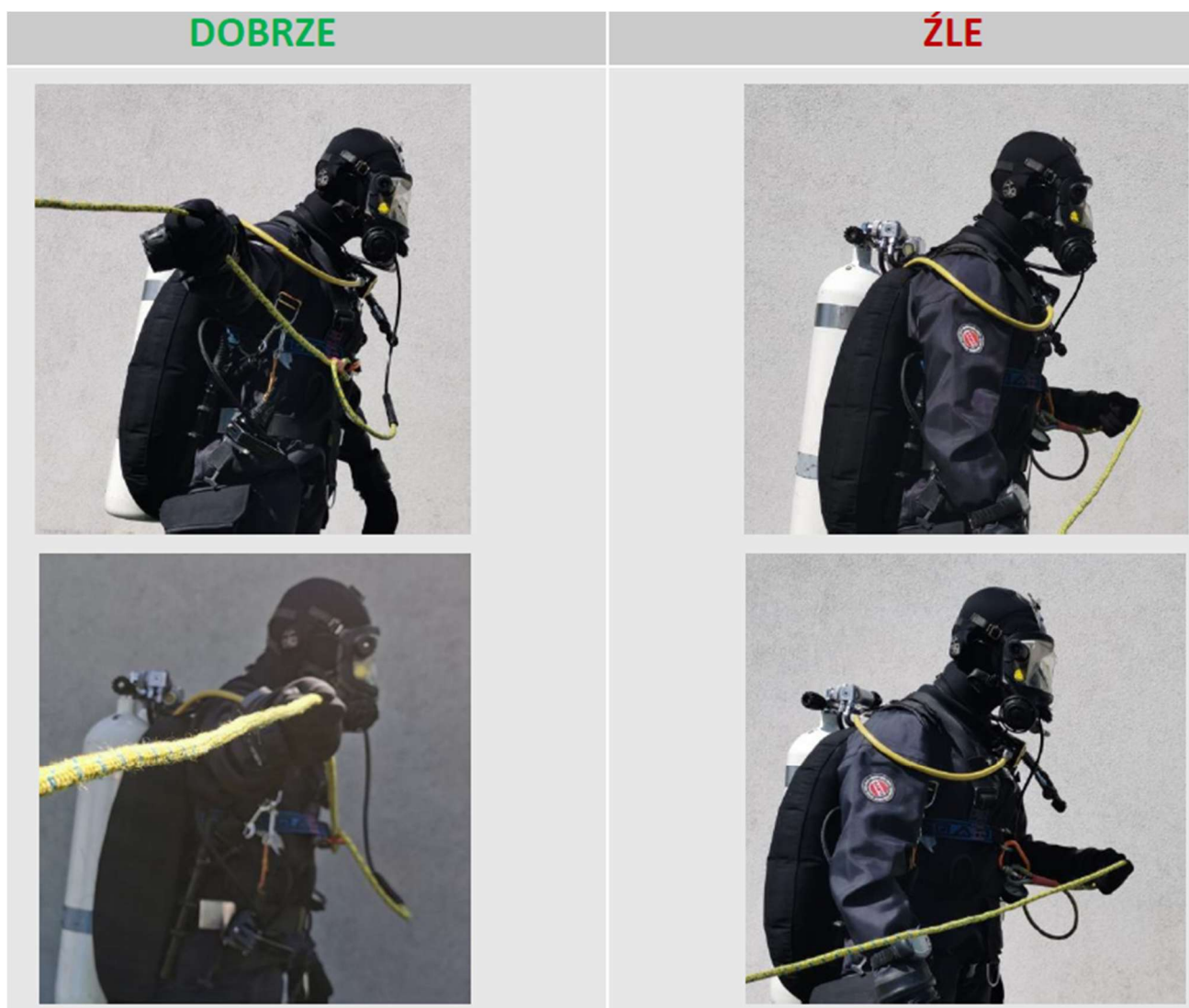
rys. 176 Instrukcja trzymania kabloliny w trakcie wahadła w prawo
