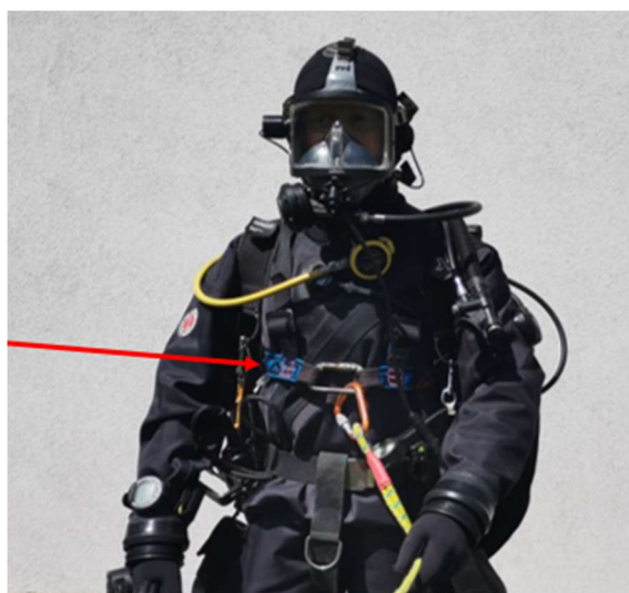
rys. 163 Prawidłowe zamocowanie liny sygnałowej/kabloliny
