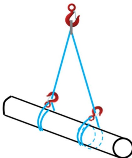
rys. 215 Instrukcja mocowania zawiesi
