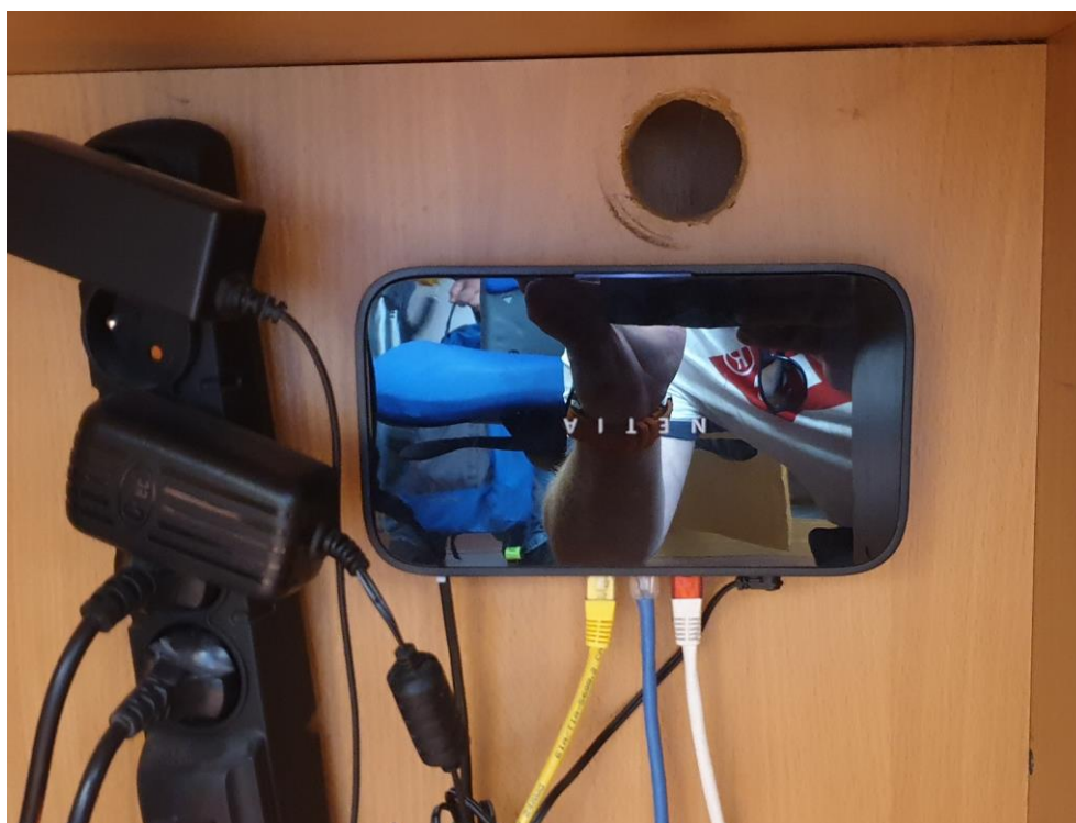
Fot. 3: Zdjęcie punktu dostępowego model Netia Spot
