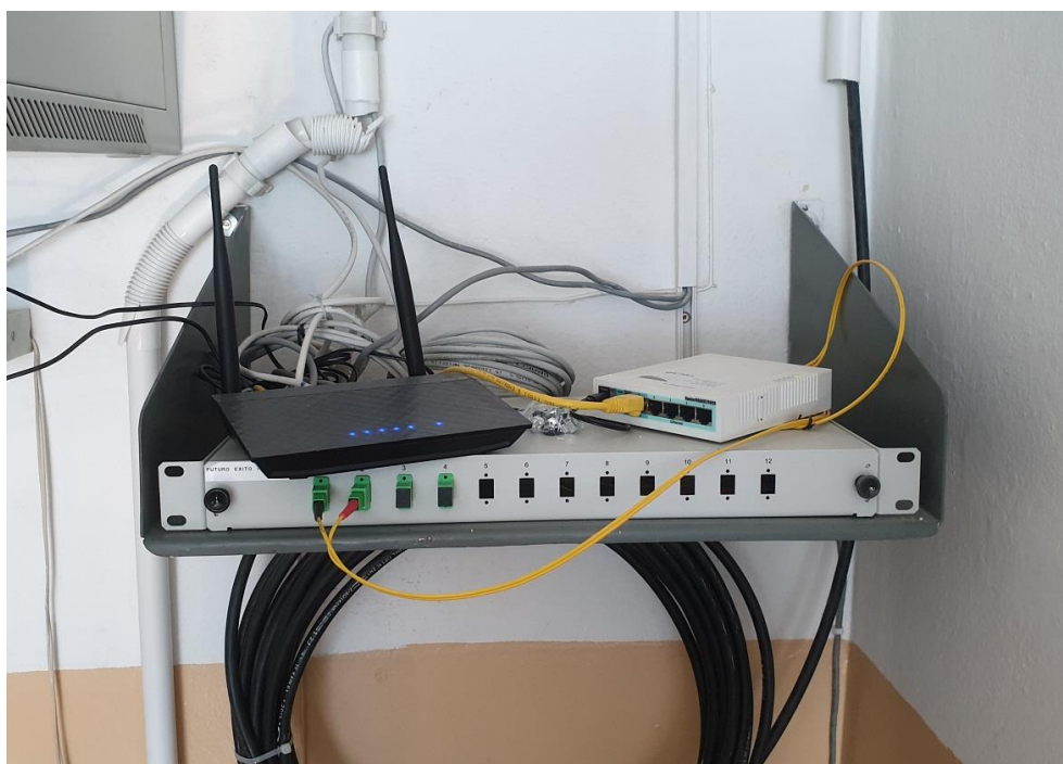
Fot. 2: Zdjęcie punktu dostępowego model RT-N12 D1
