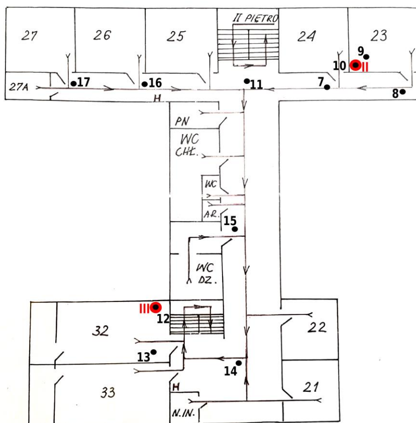
Rys. 1b: Plan rozmieszczenia punktów pomiarowych – I piętro, kolorem czerwonym oznaczono lokalizację punktów dostępowych
