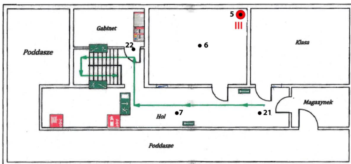
Rys. 1c: Plan rozmieszczenia punktów pomiarowych – I piętro, kolorem czerwonym oznaczono lokalizację punktu dostępowego
