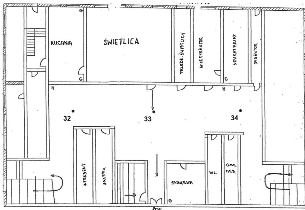
Rys. 1a: Plan rozmieszczenia punktów pomiarowych, parter
