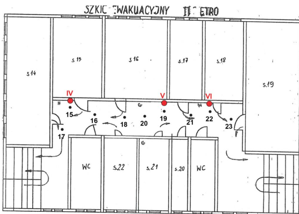
Rys. 1c: Plan rozmieszczenia punktów pomiarowych, II piętro
