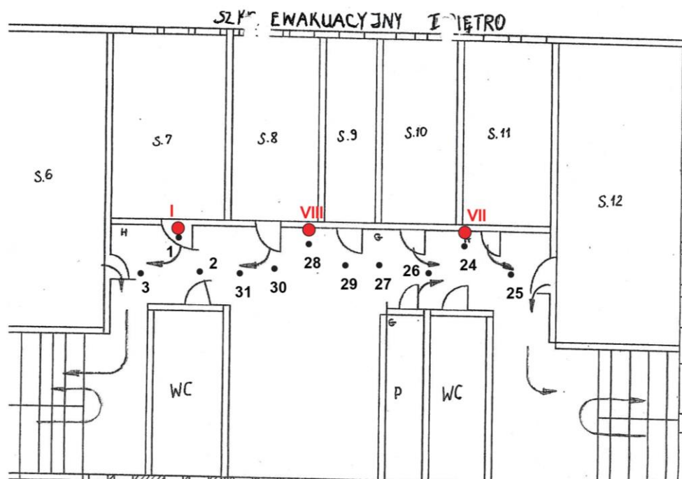
Rys. 1b: Plan rozmieszczenia punktów pomiarowych, I piętro
