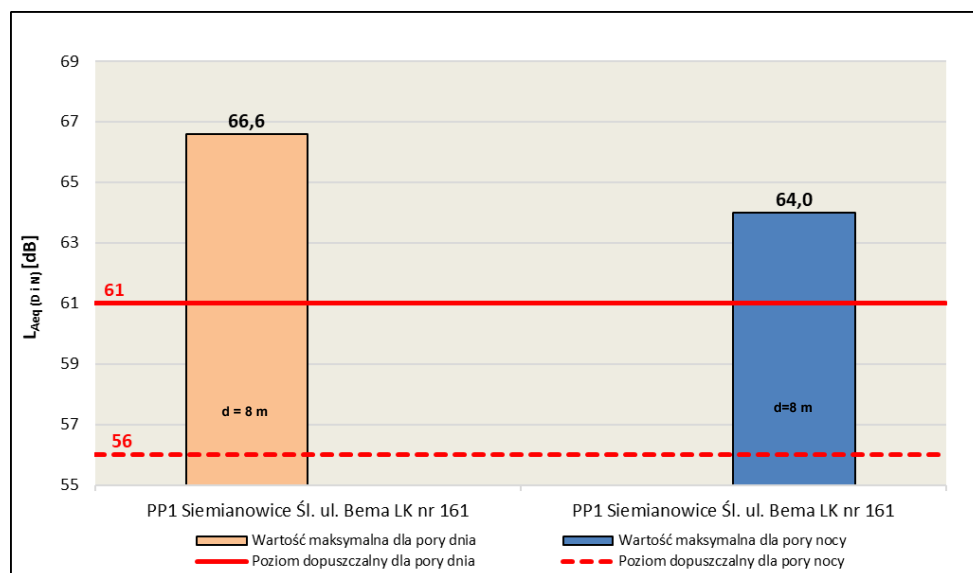
Ryc. 2. Wartość wskaźnika L AeqD i L AeqN z sesji pomiarowej dla pory dnia i nocy w badanym roku, dla rozpatrywanego punktu pomiarowego oraz jego porównanie z wartościami poziomów dopuszczalnych, Siemianowice Śląskie 2025 rok.
