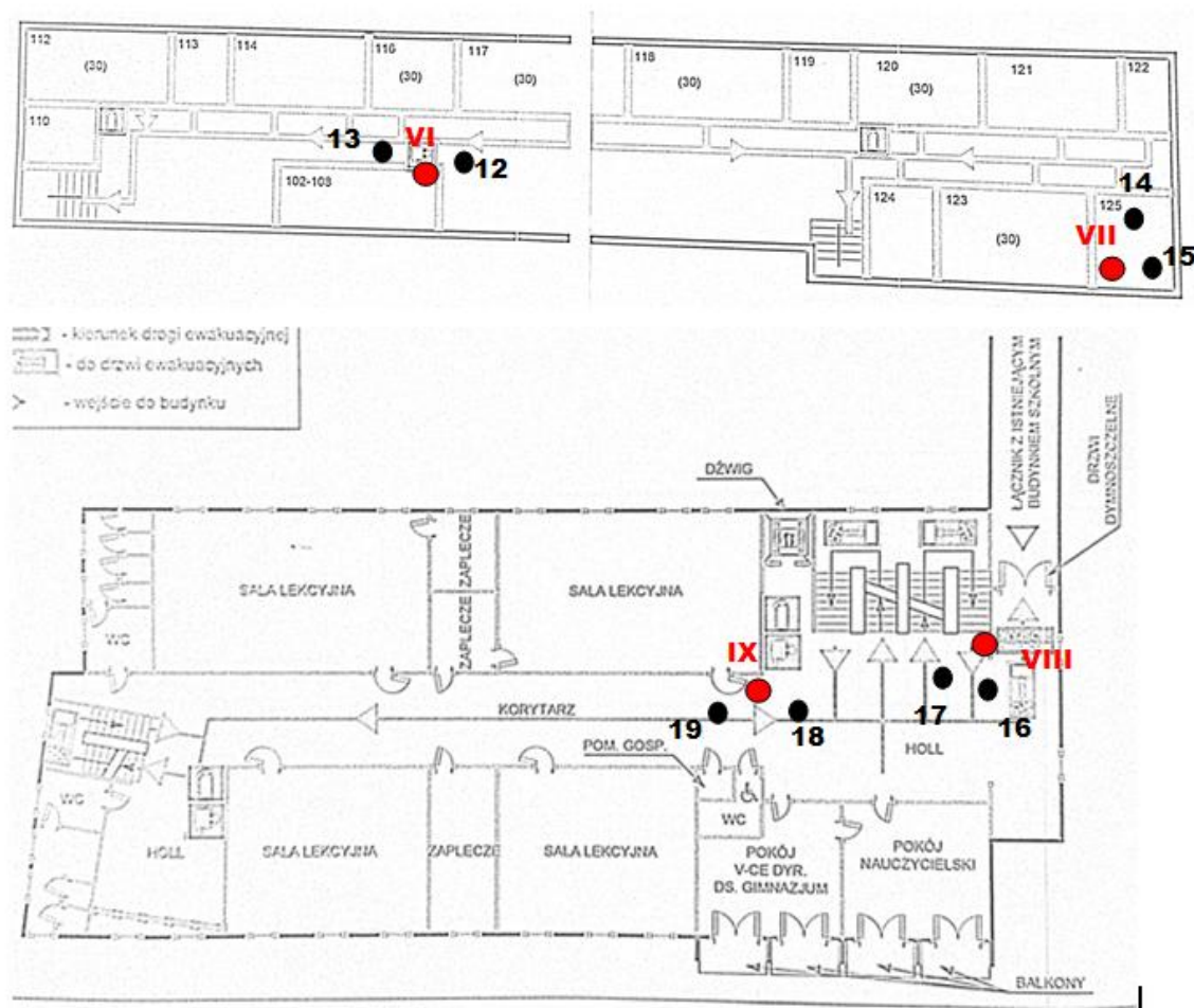
Rys. 1b: Plan rozmieszczenia punktów pomiarowych – I piętro, kolorem czerwonym oznaczono lokalizację punktów dostępnych
