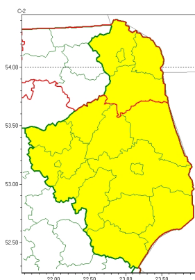
Oblodzenie 2024-01-20 12:51
