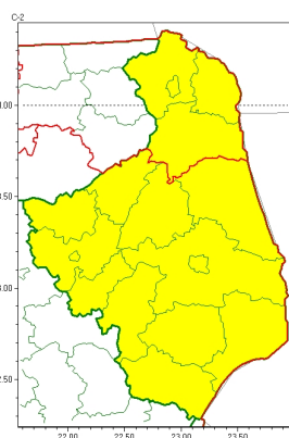
Silny wiatr 2024-01-20 12:51
