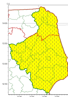
Zawieje/zamiecie śnieżne 2024-01-20 12:51
