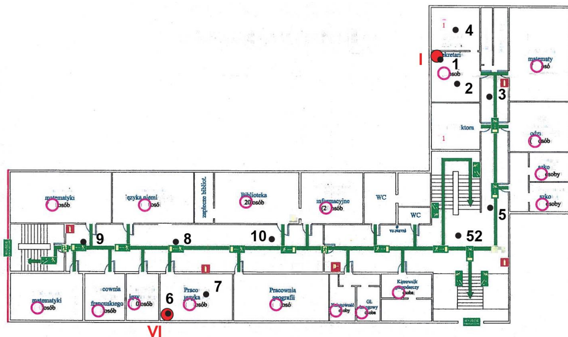
Rys. 1b: Plan rozmieszczenia punktów pomiarowych, wysoki parter, kolorem czerwonym oznaczono lokalizację punktów dostępowych
