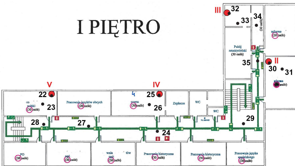
Rys. 1c: Plan rozmieszczenia punktów pomiarowych, I piętro, kolorem czerwonym oznaczono lokalizację punktów dostępowych
