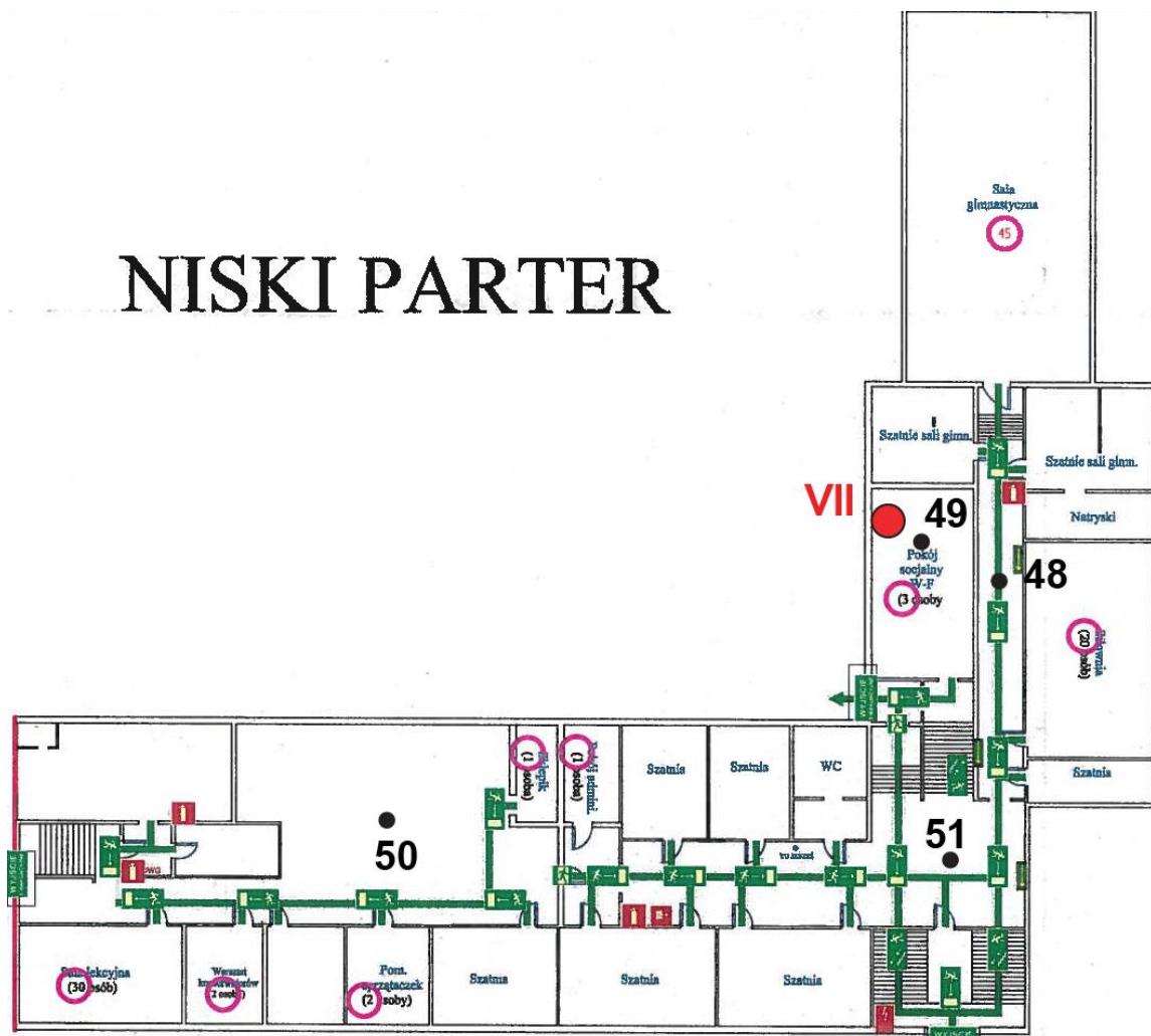
Rys. 1a: Plan rozmieszczenia punktów pomiarowych, niski parter, kolorem czerwonym oznaczono lokalizację punktów dostępowych
