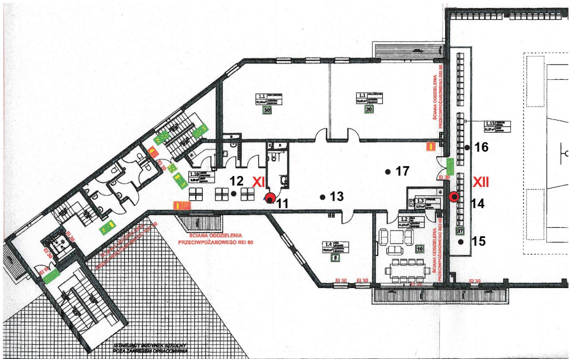
Rys. 1f: Plan rozmieszczenia punktów pomiarowych, sala sportowa – I piętro, kolorem czerwonym oznaczono lokalizację punktów dostępowych
