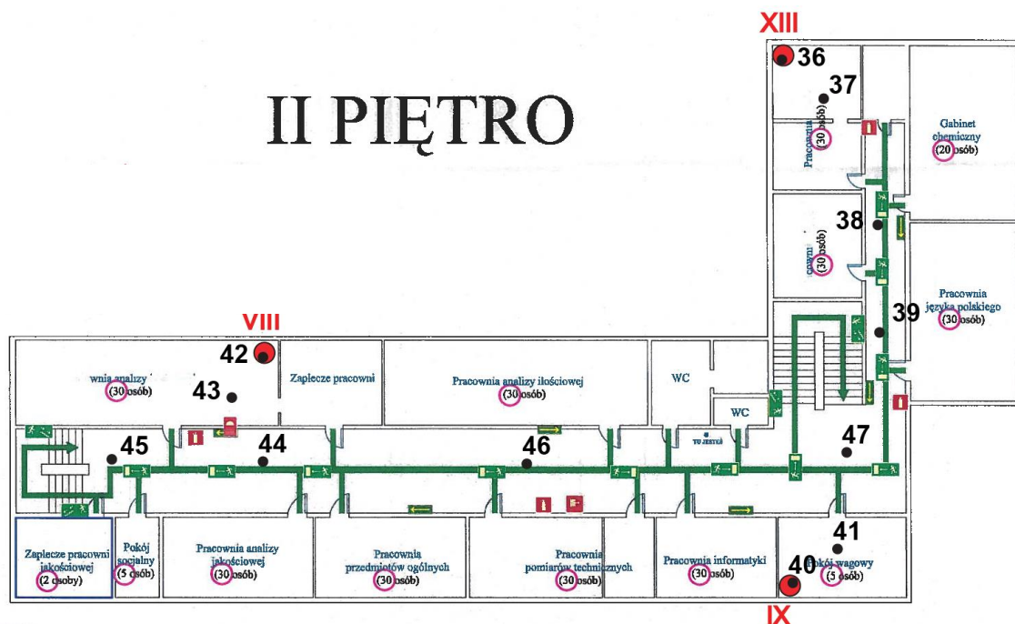
Rys. 1d: Plan rozmieszczenia punktów pomiarowych, II piętro, kolorem czerwonym oznaczono lokalizację punktów dostępowych
