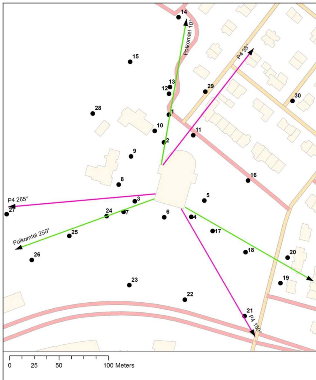
Rys. 1: Plan terenu, na którym znajdują się badane stacje bazowe
