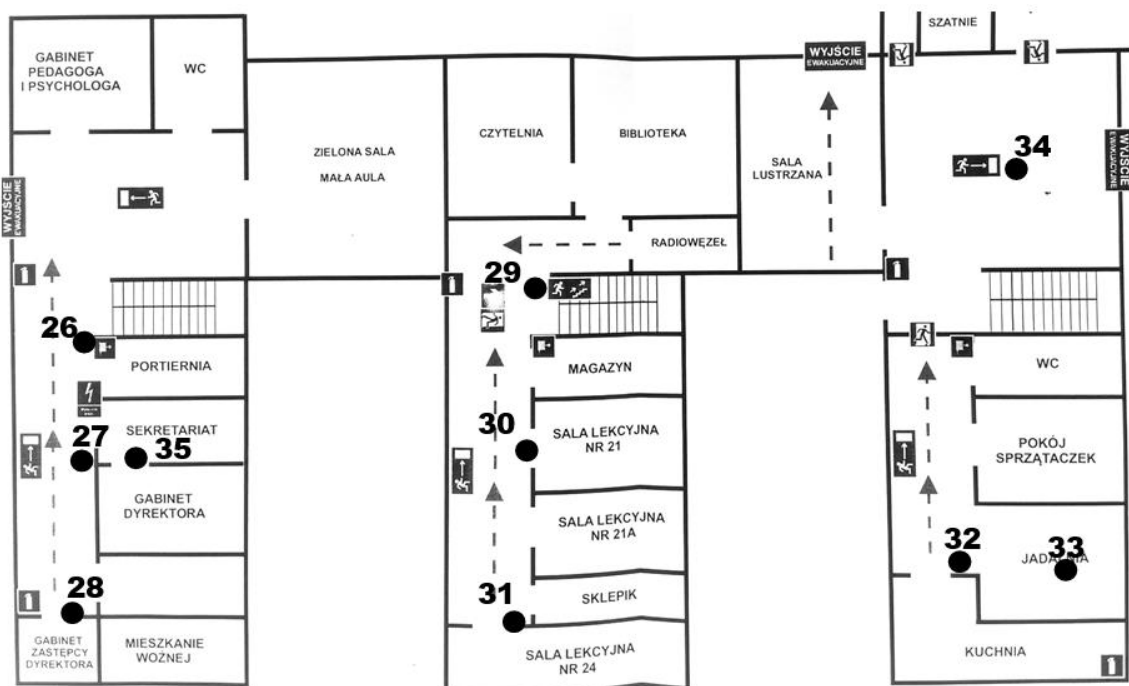
Rys. 1a: Plan rozmieszczenia punktów pomiarowych – parter
