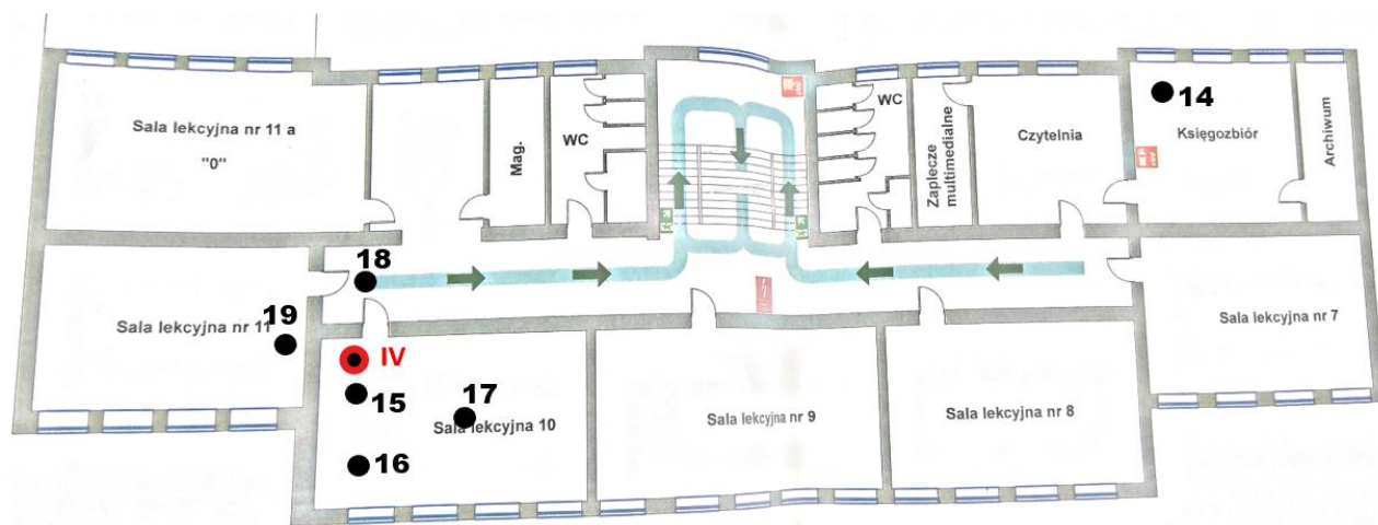
Rys. 1b: Plan rozmieszczenia punktów pomiarowych – II piętro kolorem czerwonym oznaczono lokalizację punktów dostępowych
