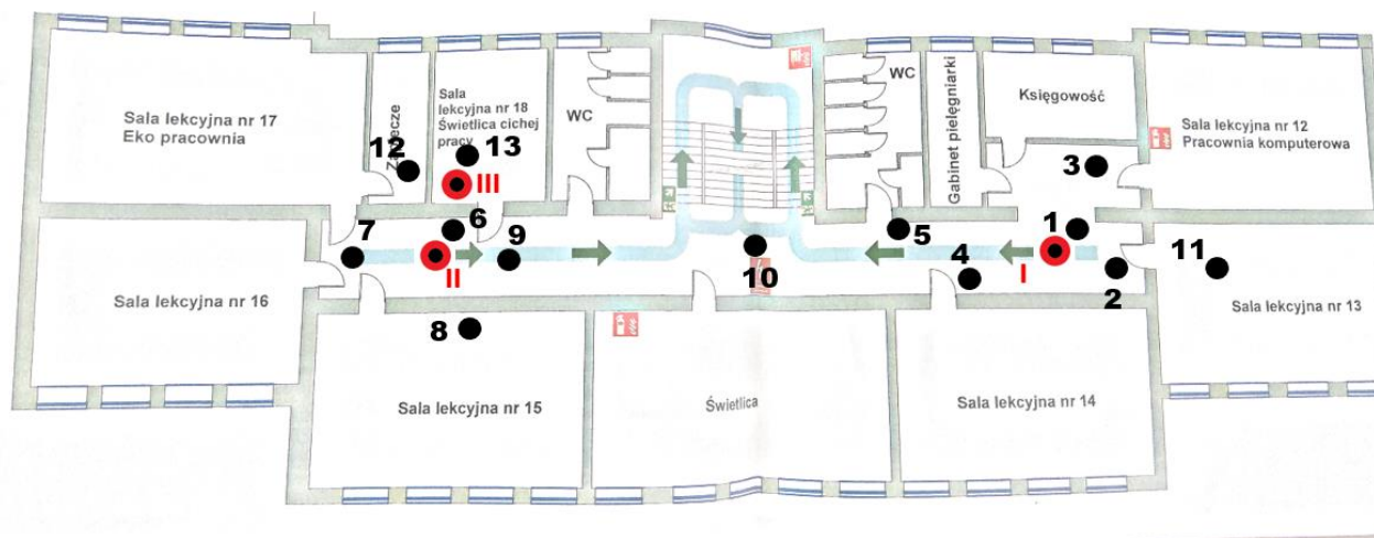
Rys. 1a: Plan rozmieszczenia punktów pomiarowych – I piętro kolorem czerwonym oznaczono lokalizację punktów dostępowych
