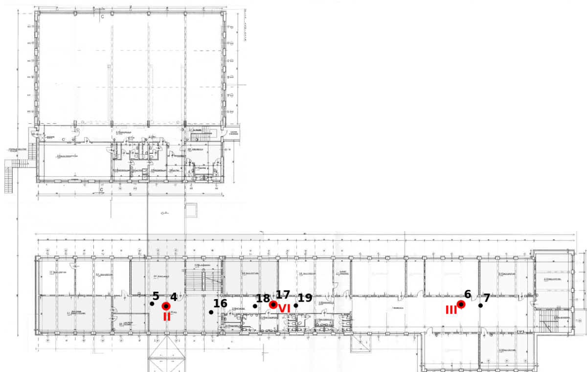
Rys. 1b: Plan rozmieszczenia punktów pomiarowych – I piętro, kolorem czerwonym oznaczono lokalizację punktów dostępowych.
