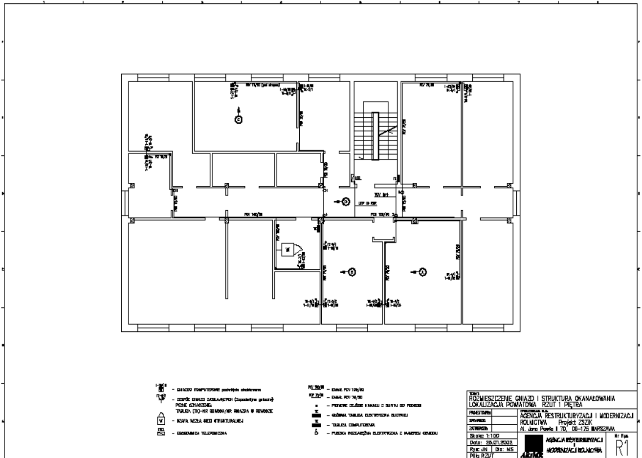
Rysunek 8: Rozmieszczenie gniazd i struktura okablowania rzut 1-szego piętra - nr R1
