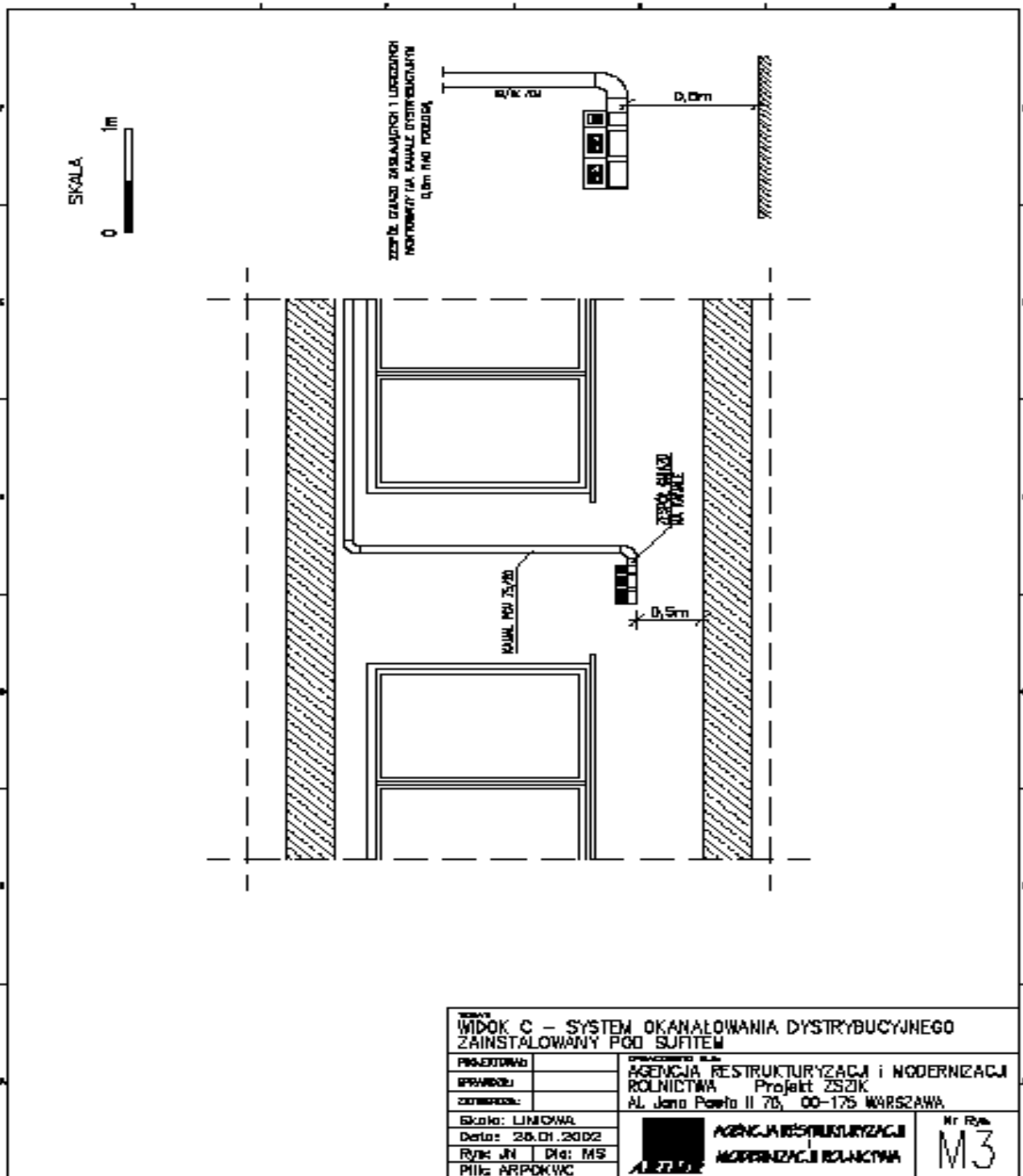
Rysunek 11: System okanałowania dystrybucyjnego zainstalowanego pod sufitem - nr M3
