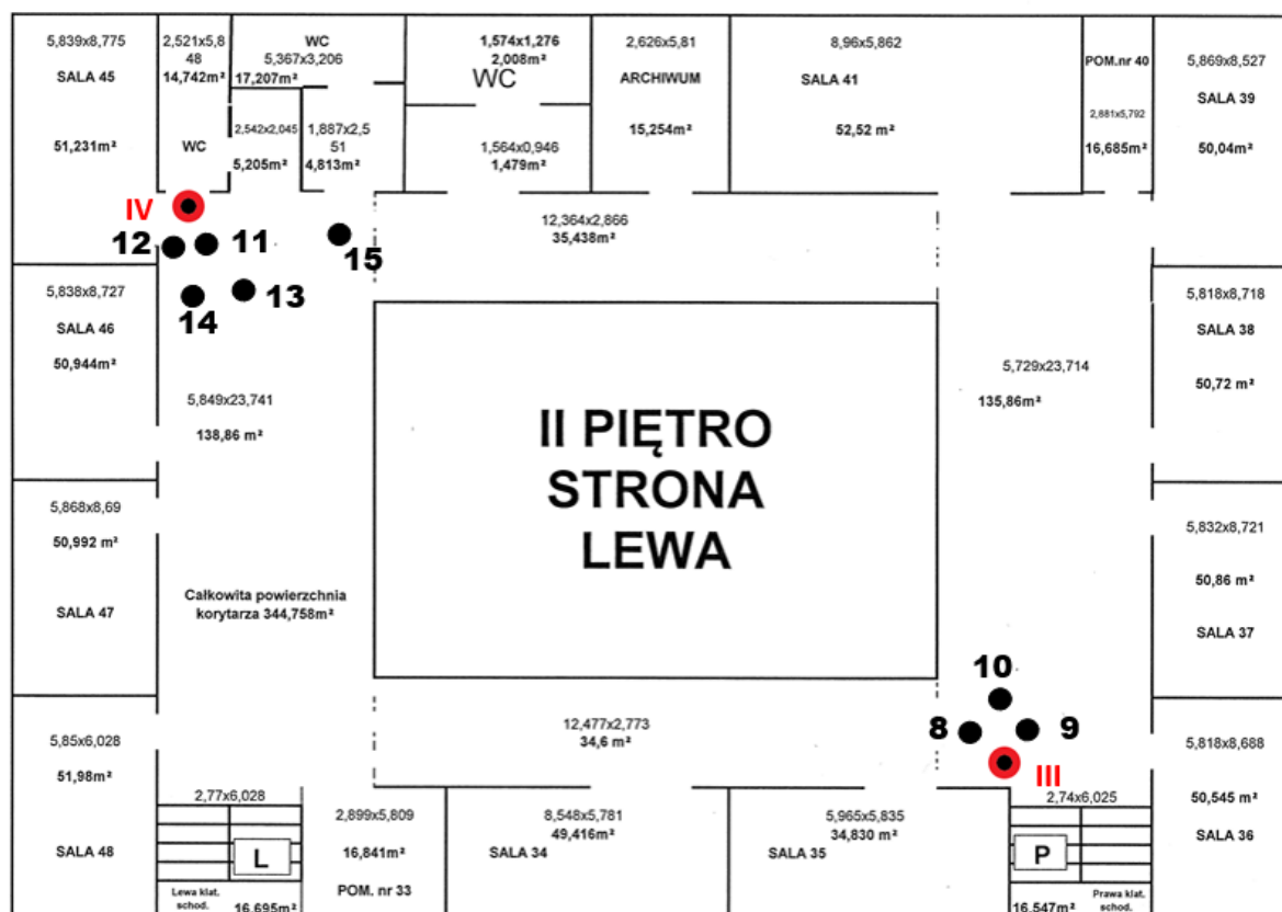
Rys. 1c: Plan rozmieszczenia punktów pomiarowych – II piętro kolorem czerwonym oznaczono lokalizację punktów dostępowych
