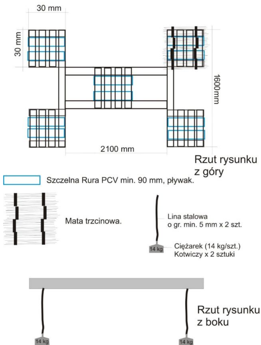
Rys. 1: Schemat platformy dla rybitwy czarnej.
