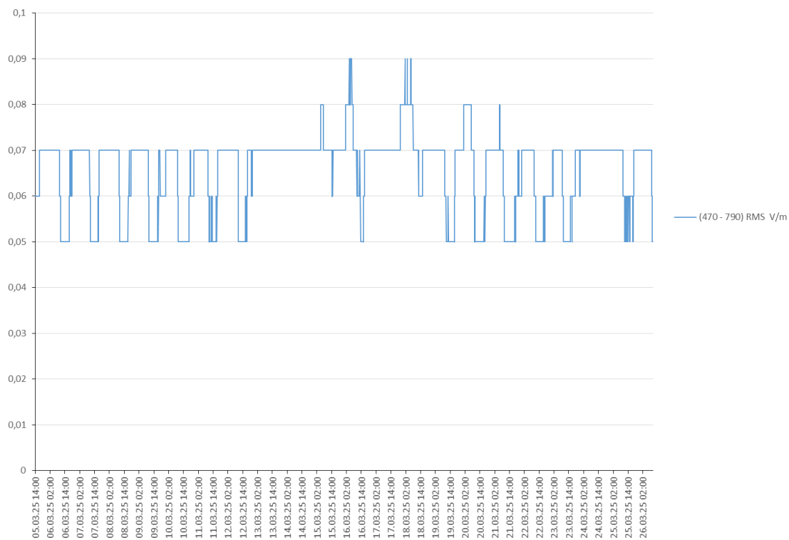
Rys. 11 Wyniki pomiarów w zakresie częstotliwości: 470,0 MHz – 790,0 MHz
