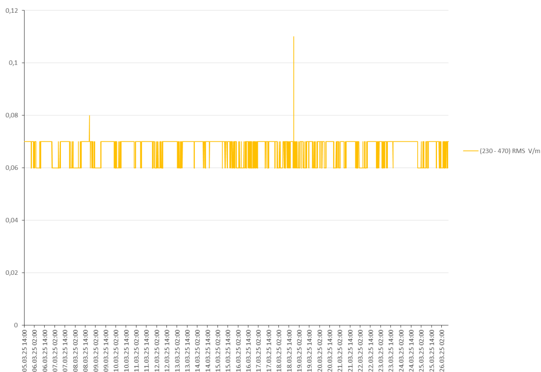
Rys. 10 Wyniki pomiarów w zakresie częstotliwości: 230,0 MHz – 470,0 MHz
