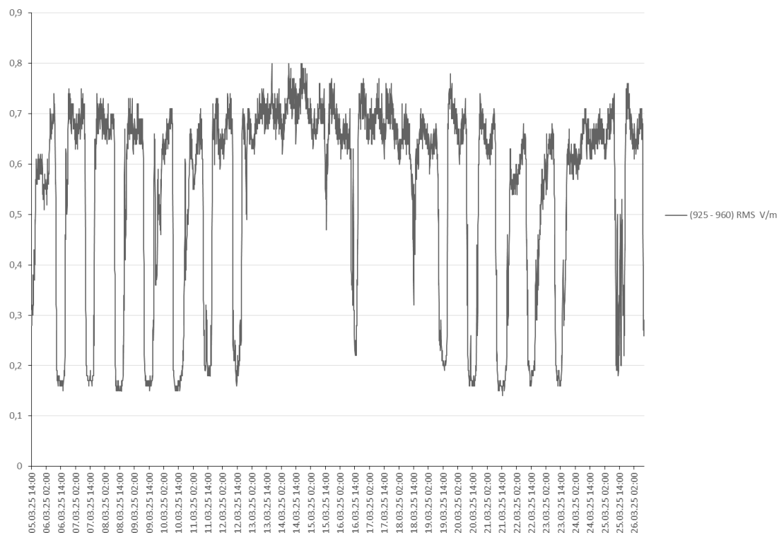
Rys. 15 Wyniki pomiarów w zakresie częstotliwości: 925,0 MHz – 960,0 MHz
