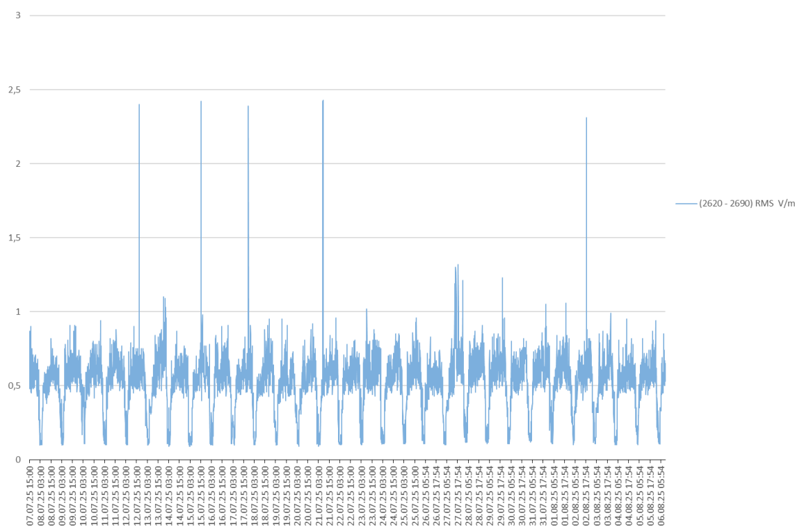
Rys. 45 Wyniki pomiarów w zakresie częstotliwości: 2620,0 MHz – 2690,0 MHz
