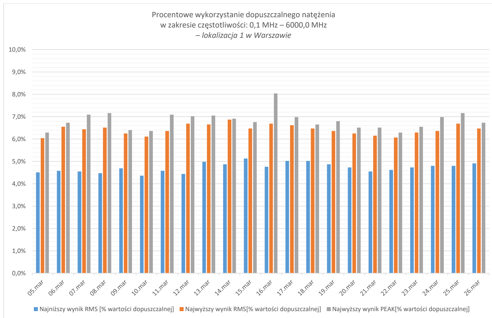
Rys. 26 Procentowe wykorzystanie dopuszczalnego natężenia w zakresie częstotliwości: 0,1 MHz – 6000,0 MHz – lokalizacja 1
