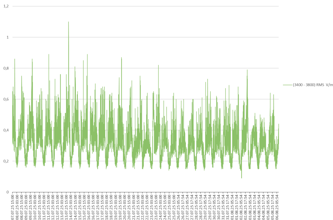
Rys. 46 Wyniki pomiarów w zakresie częstotliwości: 3400,0 MHz – 3800,0 MHz
