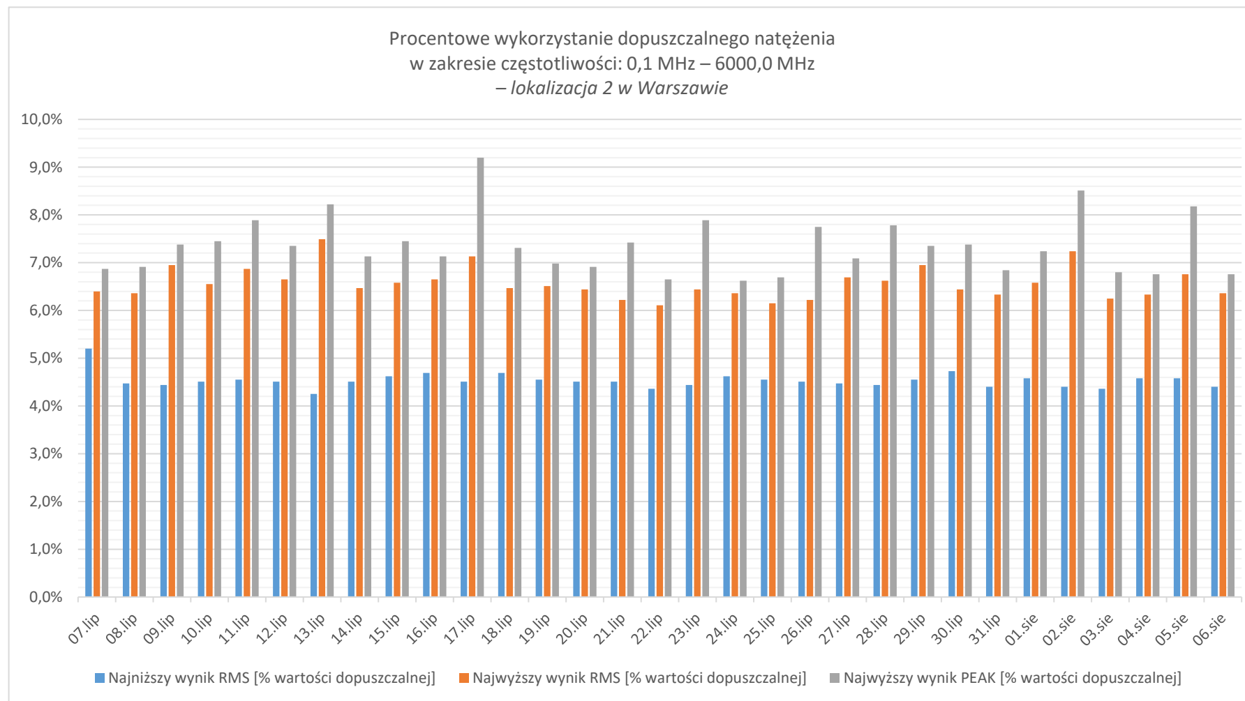
Rys. 48 Procentowe wykorzystanie dopuszczalnego natężenia w zakresie częstotliwości: 0,1 MHz – 6000,0 MHz – lokalizacja 2
