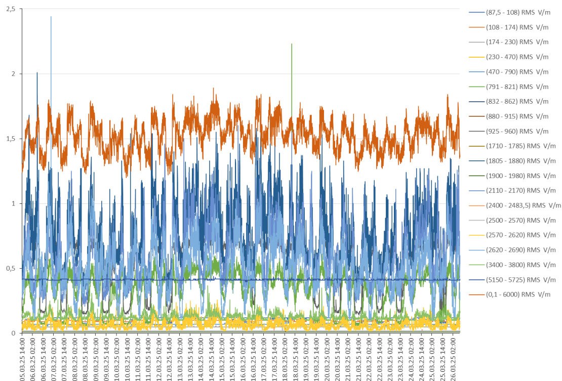
Rys. 5 Wyniki pomiarów dla 20 podzakresów częstotliwości – lokalizacja 1
