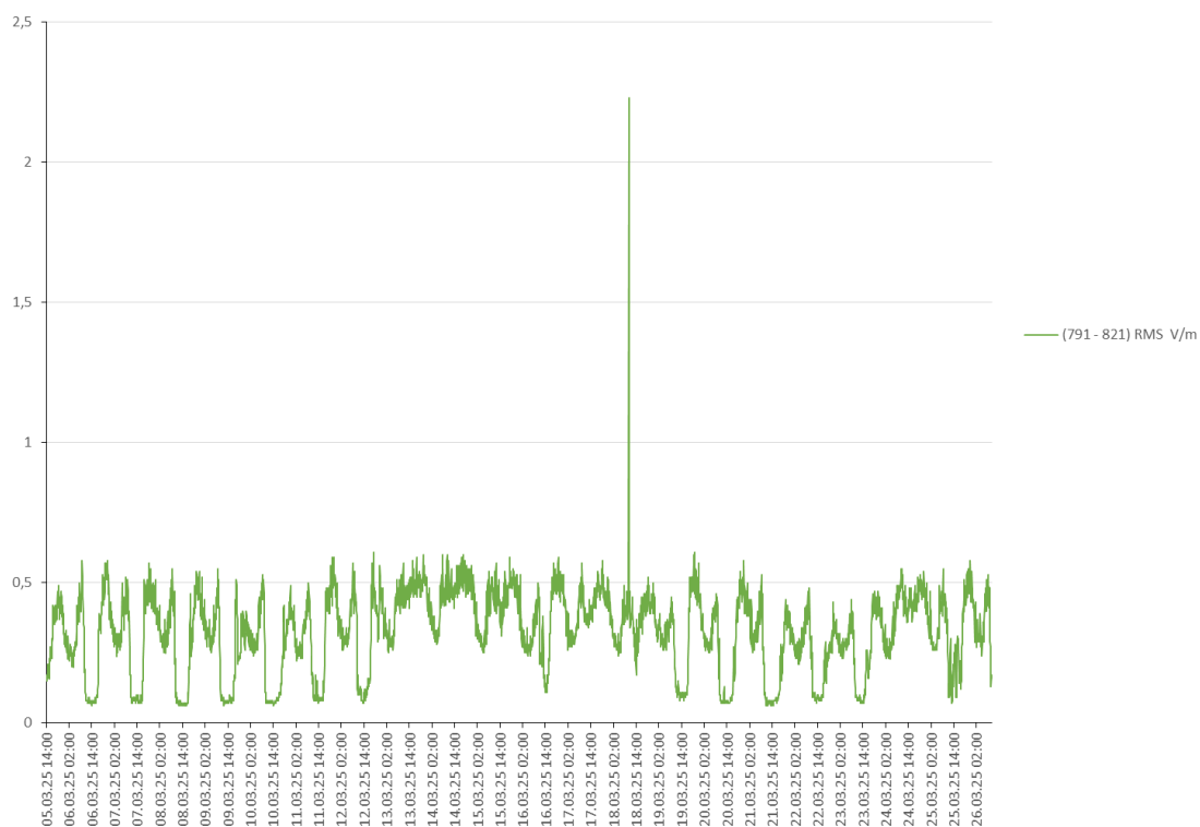
Rys. 12 Wyniki pomiarów w zakresie częstotliwości: 791,0 MHz – 821,0 MHz
