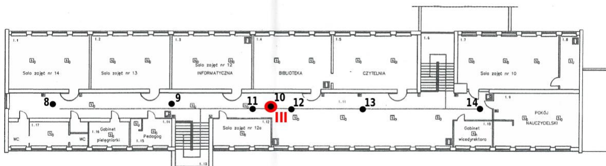
Rys. 1b: Plan rozmieszczenia punktów pomiarowych – parter, kolorem czerwonym oznaczono lokalizację punktów dostępowych.
