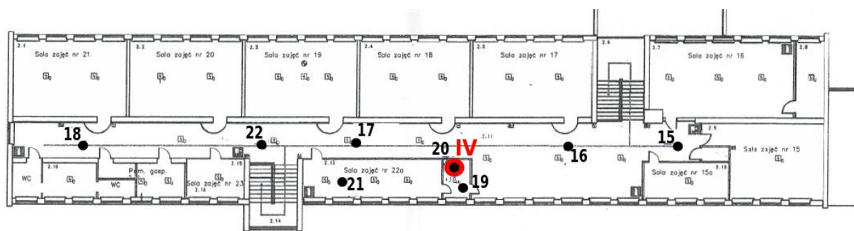
Rys. 1d: Plan rozmieszczenia punktów pomiarowych – II piętro, kolorem czerwonym oznaczono lokalizację punktów dostępowych.
