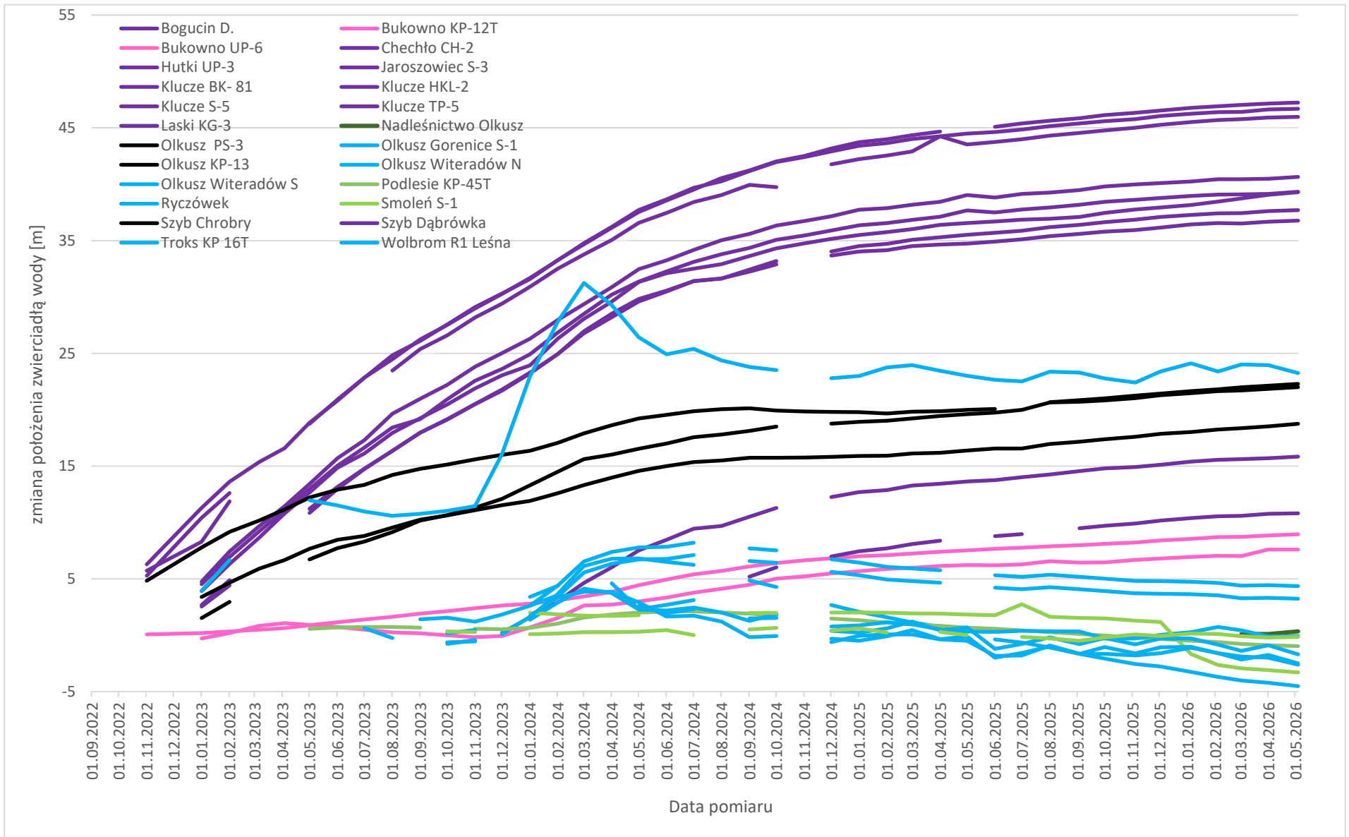
Ryc. 10. Wykresy położenia zwierciadła wody w punktach obserwacyjno-badawczych w podziale na charakterystykę odbudowywania się zwierciadła wody (lokalizacja punktów przedstawiona na Ryc. 6)
