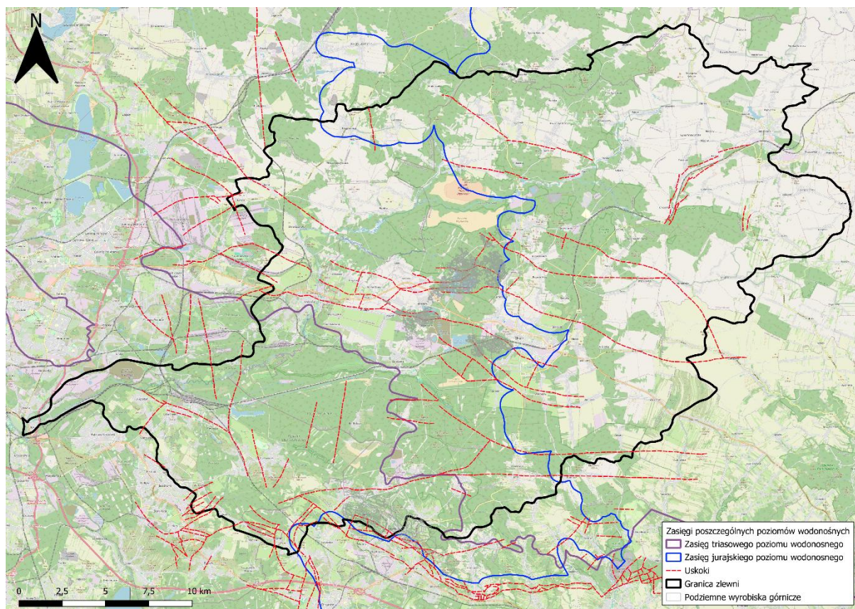
Ryc. 7. Zasięg występowania triasowego i jurajskiego poziomu wodonośnego
