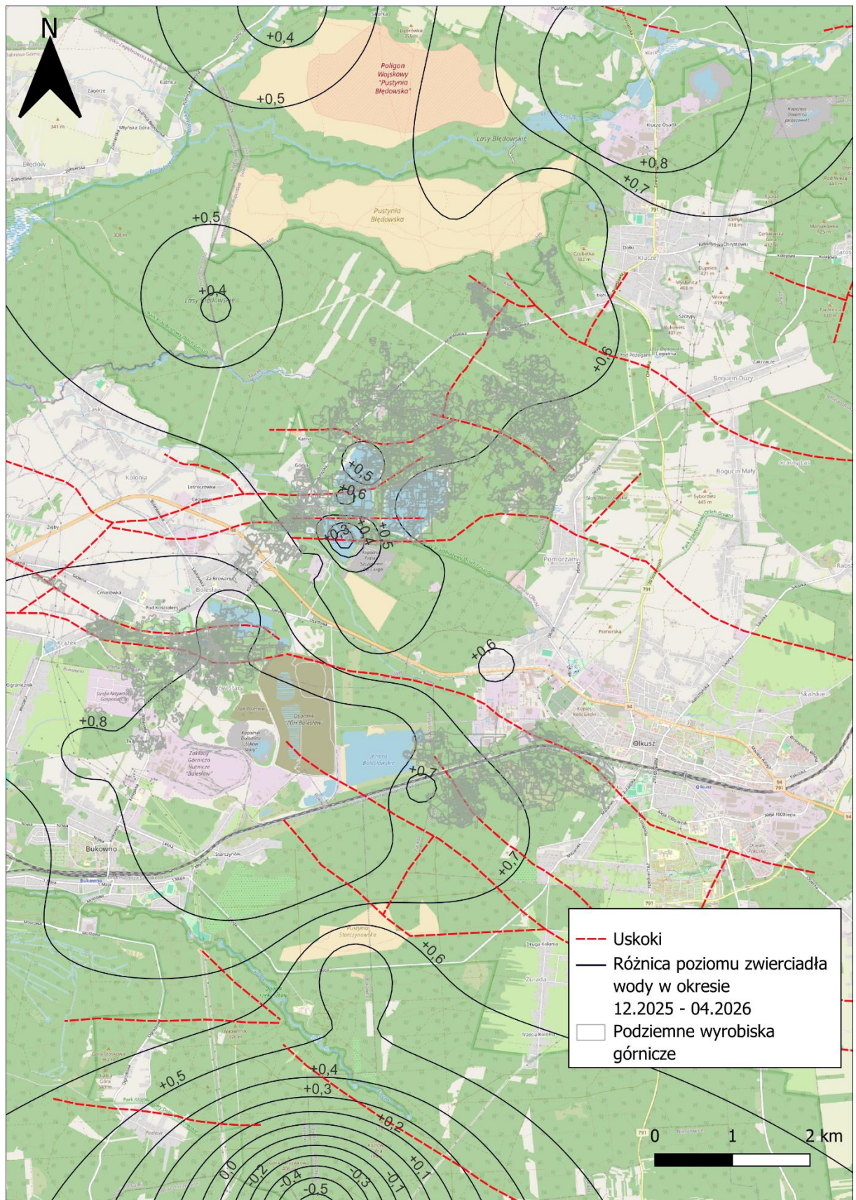
Ryc. 81. Zmiana położenia zwierciadła wody w poziomie triasowym w okresie od grudnia 2025 r. do kwietnia 2026 r.
