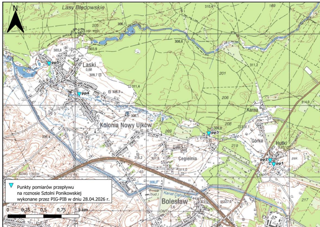
Ryc. 14. Lokalizacja punktów pomiaru przepływu na roznosie Sztolni Ponikowskiej
