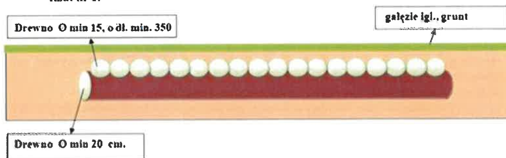
Rzut nr 1.
