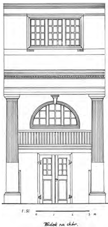
13. Widok na chór muzyczny i wejście do kruchty, rys. J. Górak
