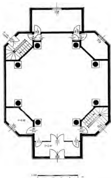
Plan przyziemia.
