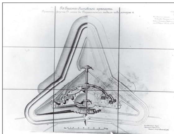
9. Koroszczyn, fort „O”, rzut planu fortu proj. N.A. Bujnickiego, fot. archiwum WUOZ Lublin/Biała Podl.
