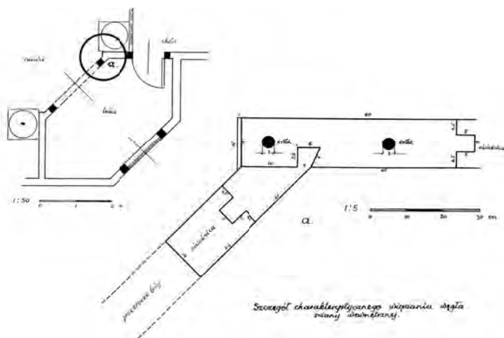
12. Szczegół charakterystycznego wiązania węgła, rys. J. Górak
