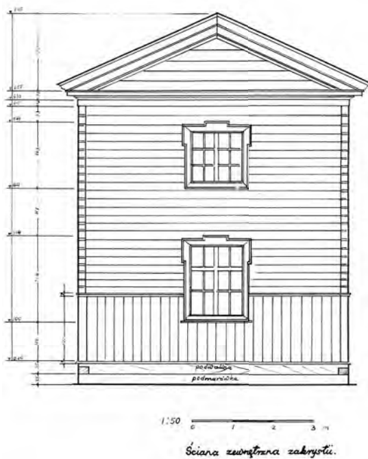
14. Ściana północna zakrystii z uszkowymi obramieniami okien, stan przed 1980 r.
