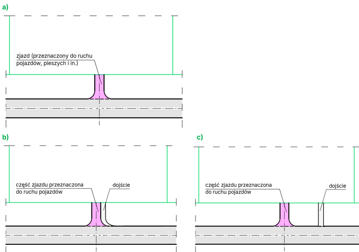
Rys. 4.2.1. Sposoby rozwiązania dostępu do drogi przez zjazd zwykły: a) rozwiązanie standardowe; b) i c) rozwiązania alternatywne, dopuszczalne w trudnych warunkach
