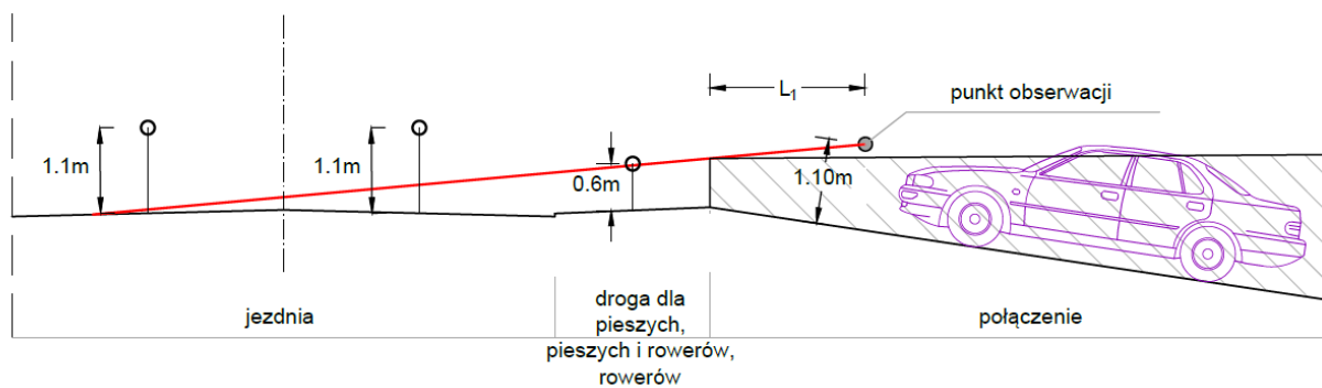
Rys. 7.6. Schemat wyznaczenia pola widoczności w płaszczyźnie poziomej i pionowej – przypadek II według rys. 7.4
