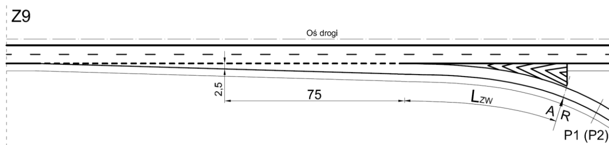
Rys. 9.3.1.2. Schemat typowego rozwiązania wyjazdu z kierunkowym pasem wyłączenia
