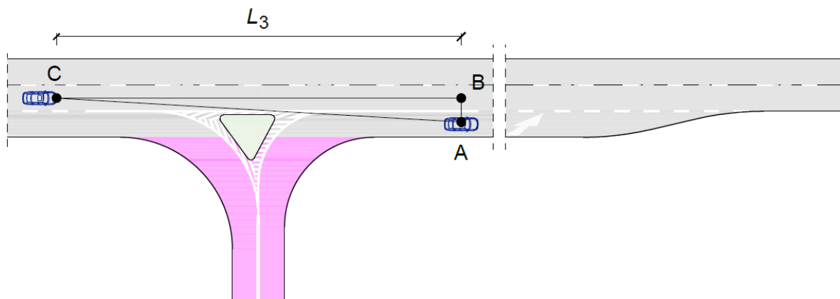
Rys. 7.3. Schemat wyznaczenia pola widoczności na połączeniu z pasem włączania
