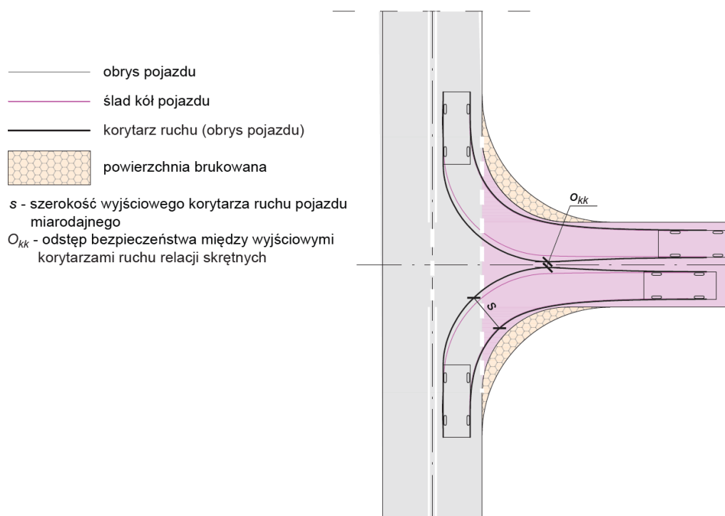
Rys. 4.4.1. Przykład sprawdzania przejeźdźności dla dwóch relacji skrzyżnych na połączeniu
