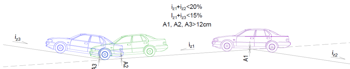
Rys. 8.3.1. Kształtowanie pochyłeń podłużnych zjazdu przy dużych spadkach
