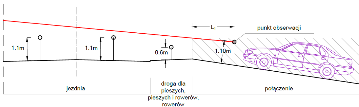
Rys. 7.5. Schemat wyznaczenia pola widoczności w płaszczyźnie poziomej i pionowej – przypadek I według rys. 7.4
