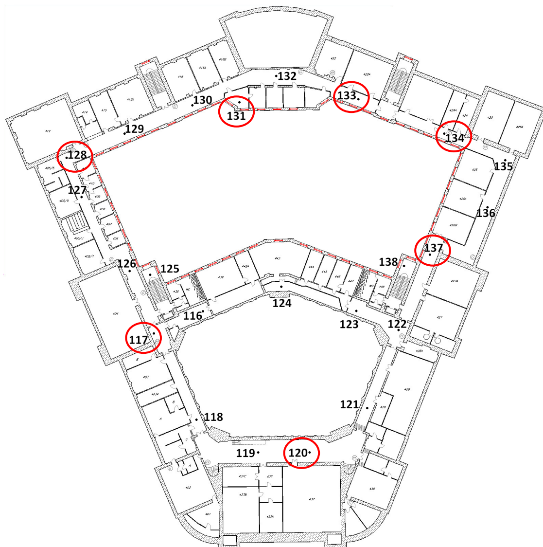
Rys. 6: Gmach Główny, IV piętro, kolorem czerwonym oznaczono piony pomiarowe pod punktami dostępowymi
