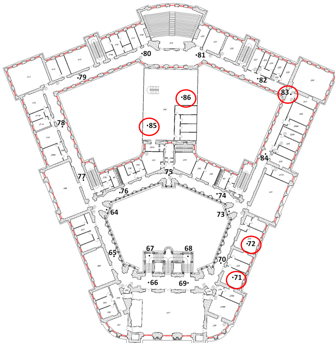
Rys. 4: Gmach Główny, II piętro, kolorem czerwonym oznaczono pionowy pomiarowe pod punktami dostępowymi
