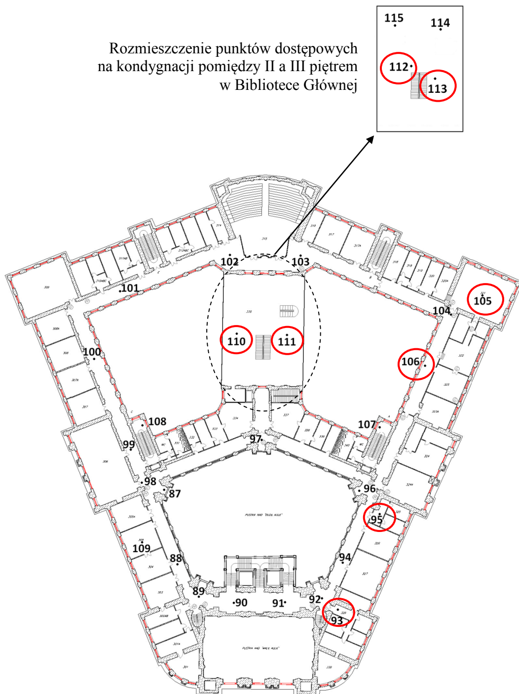
Rys. 5: Gmach Główny, III piętro, kolorem czerwonym oznaczono pionys pomiarowe pod punktami dostępowymi
