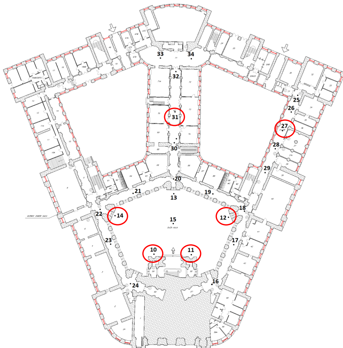
Rys. 2: Gmach Główny, parter, kolorem czerwonym oznaczono pionowy pomiarowe pod punktami dostępowymi
