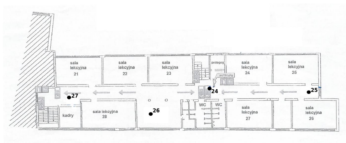
Rys. 1f: Plan rozmieszczenia punktów pomiarowych – I piętro, bryła C
