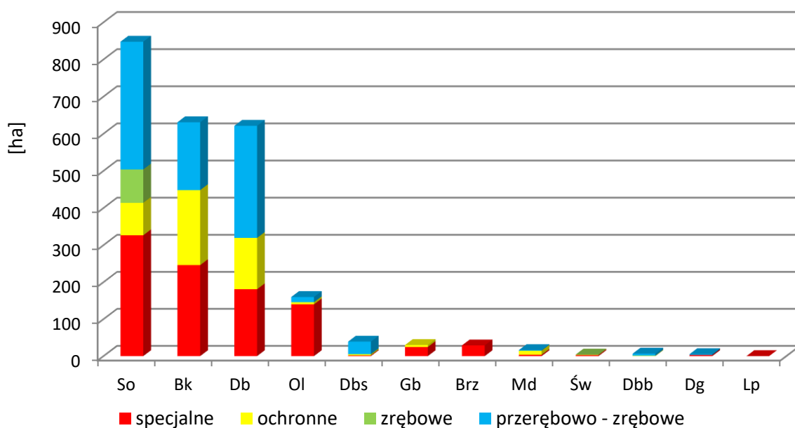
Wykres 12. Powierzchnia gatunków panujących w drzewostanach ponad 100-letnich wg gospodarstw w Nadleśnictwie
