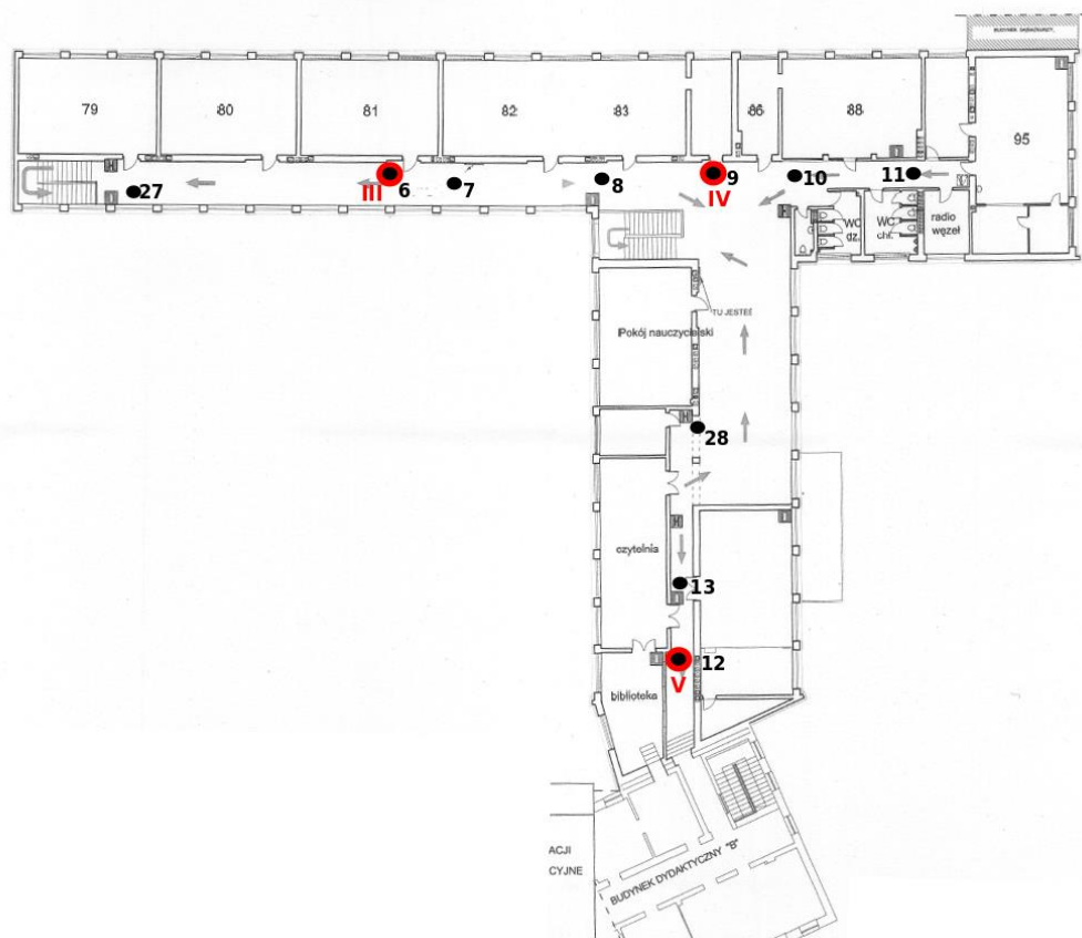
Rys. 1c: Plan rozmieszczenia punktów pomiarowych – I piętro, część I, kolorem czerwonym oznaczono lokalizacje punktów dostępowych
