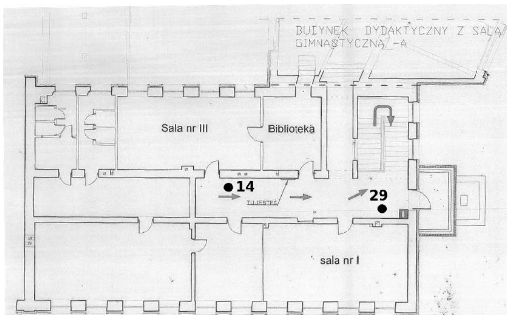
Rys. 1d: Plan rozmieszczenia punktów pomiarowych – I piętro, część II
